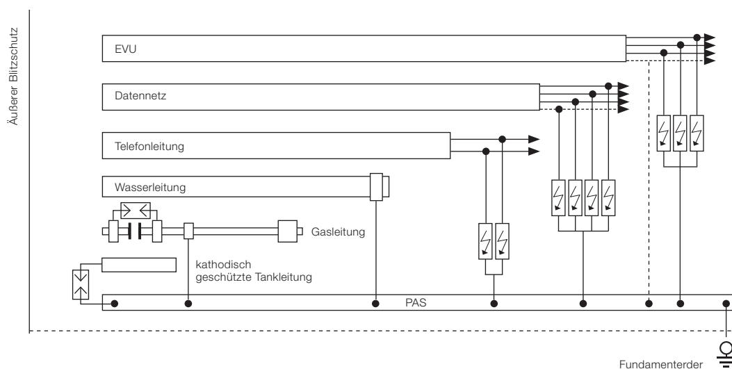
Abbildung 10: Ableitpfade in einem Gebäude mit äußerer Blitzschutzanlage
