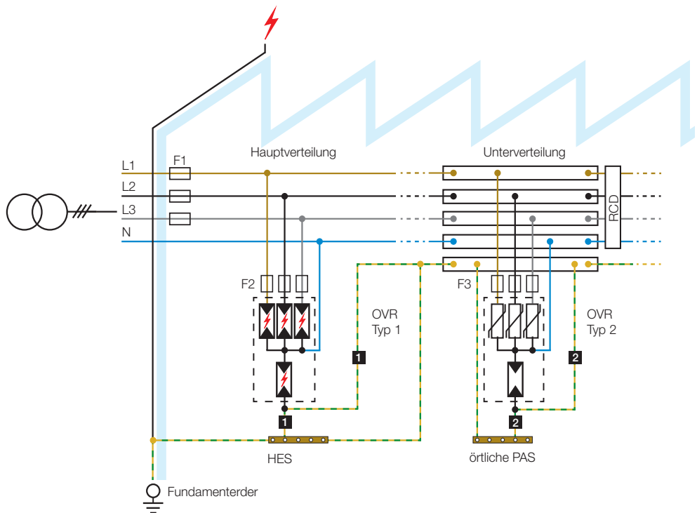
Abbildung 3: Einsatz von Blitzstrom- und Überspannungsableitern in einem Industriegebäude mit einem TT-System
