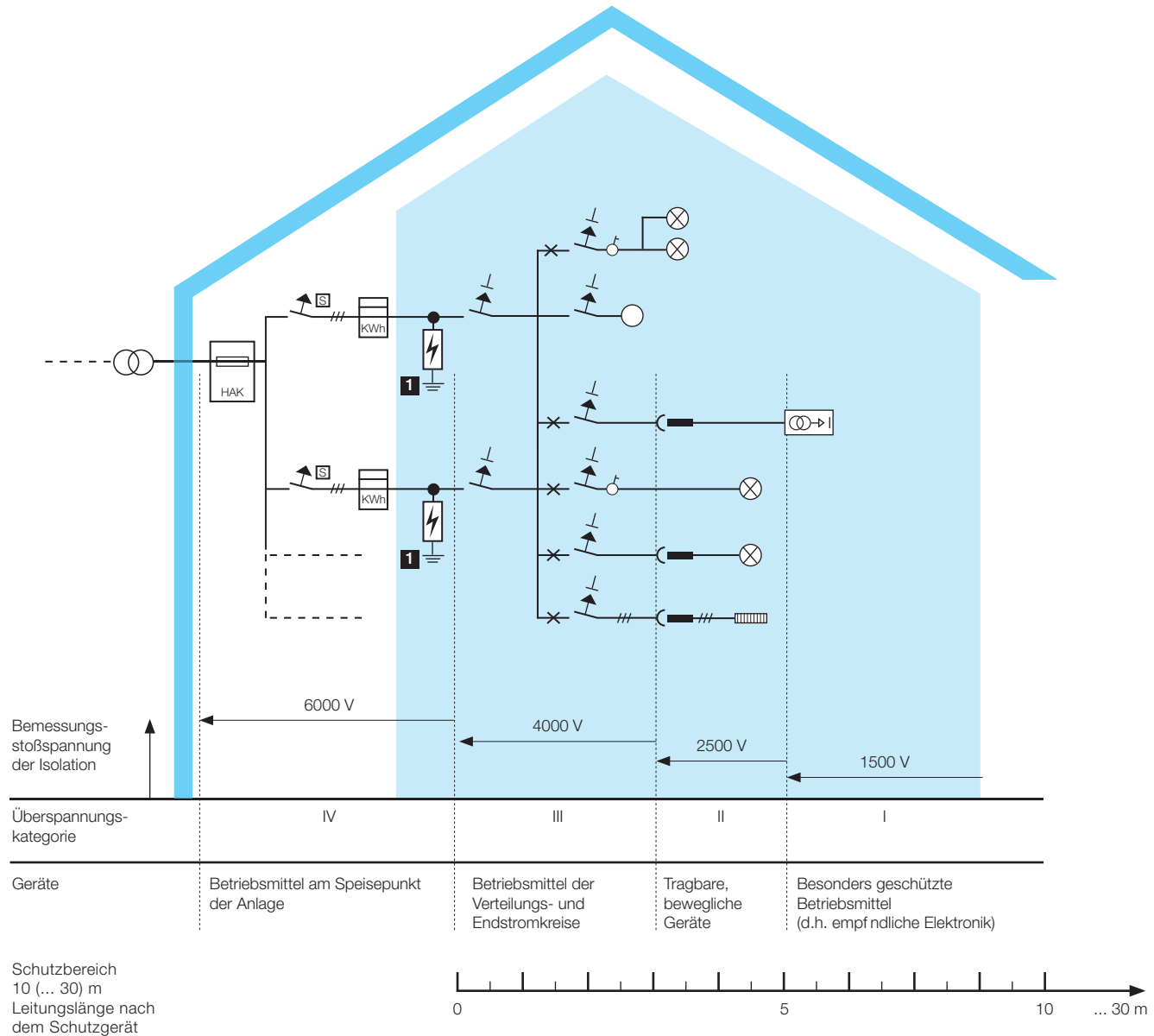
Abbildung 18: Schutzbereich eines Typ 1+2 Ableiters (OVR T1+2) im 230/400 V AC Netz
