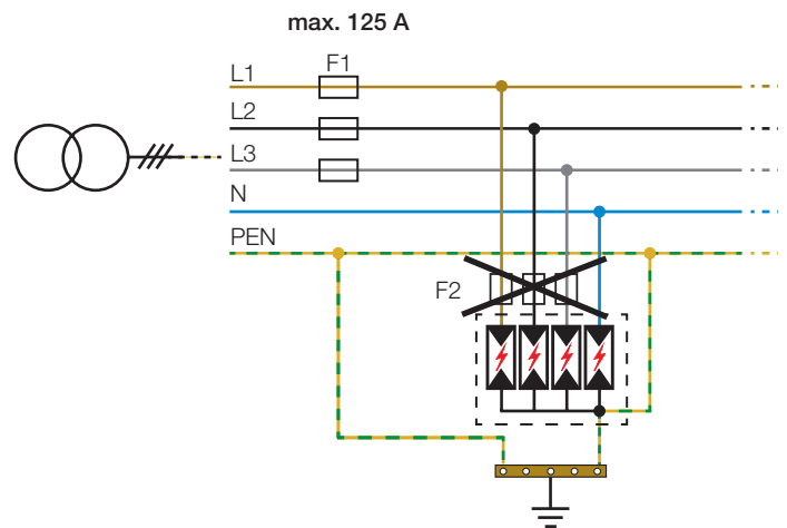
Abbildung 14: Vorsicherung als Backup-Schutz für Überspannungsableiter nicht notwendig
