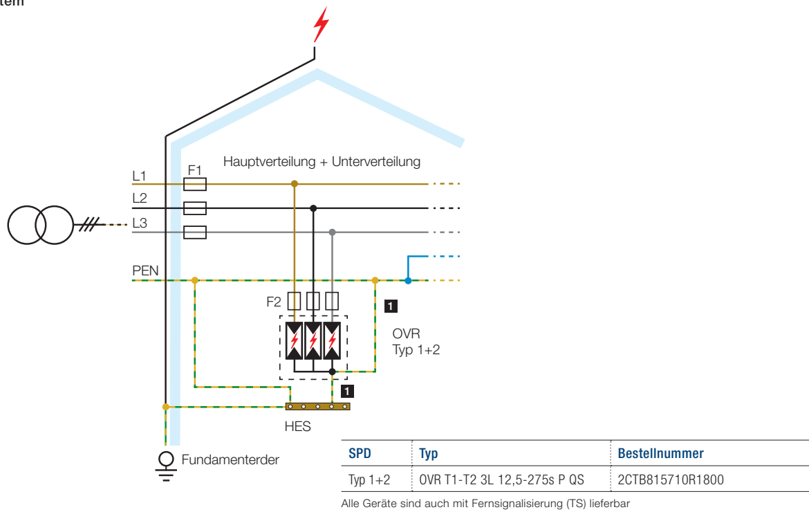
Abbildung 5: Einsatz von kombinierten Blitzstrom- und Überspannungsableitern in einem Wohngebäude mit äußerer Blitzschutzanlage und mit einem TN-C-S-System
