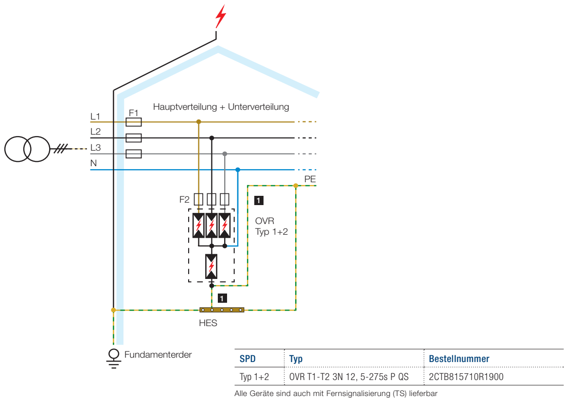
Abbildung 6: Einsatz von kombinierten Blitzstrom- und Überspannungsableitern in einem Wohngebäude mit äußerer Blitzschutzanlage und mit einem TT-System
