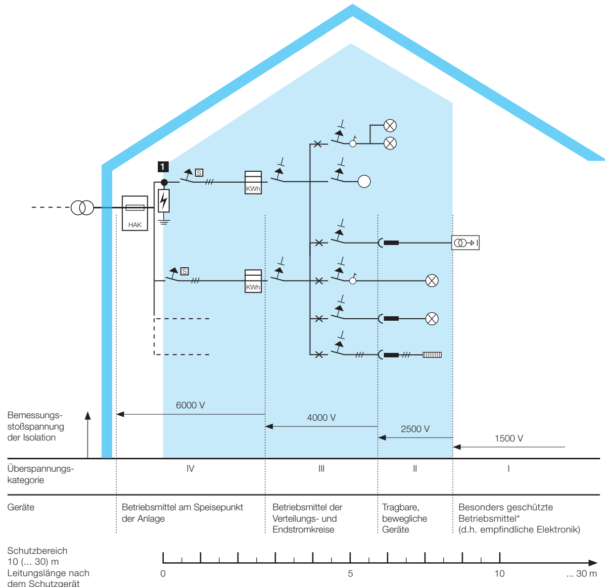
Abbildung 17: Schutzbereich eines Typ 1 Ableiters (OVR T1)
