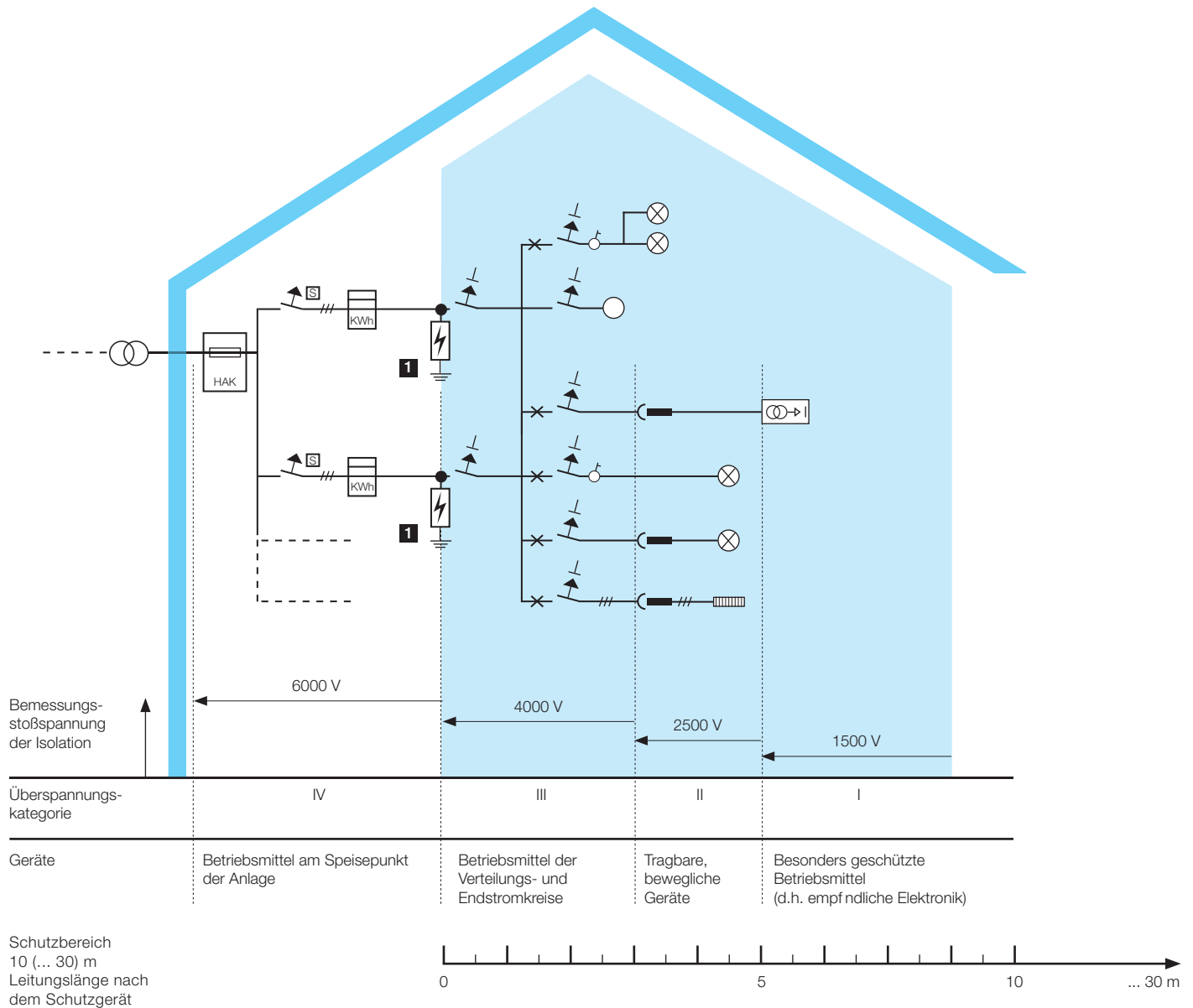
Abbildung 19: Schutzbereich eines Typ 2 Ableiters (OVR T2)
