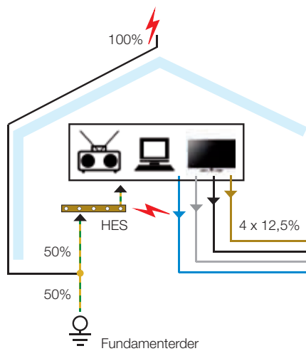
Abbildung 12: Dimensionierung des notwendigen Ableitvermögens bei einem Typ 1 Blitzstromableiter in Blitzschutzklasse (LPL) I, III und IV nach dem vereinfachten Verfahren
