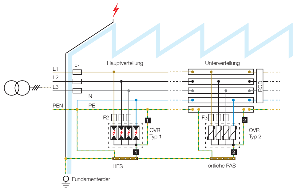
Abbildung 1: Einsatz von Blitzstrom- und Überspannungsableitern in einem Industriegebäude mit einem TN-S-System
