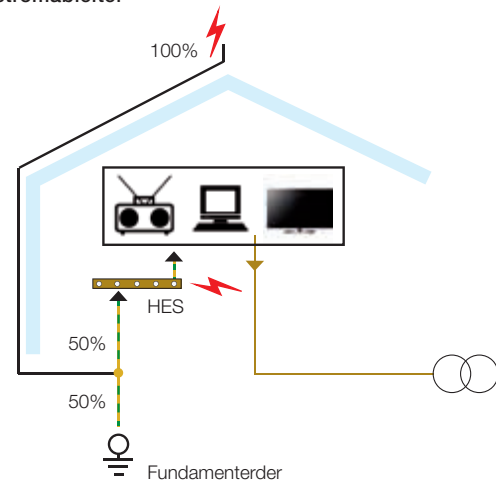
Abbildung 11: Vereinfachtes Verfahren zur Dimensionierung der Typ 1 Blitzstromableiter
