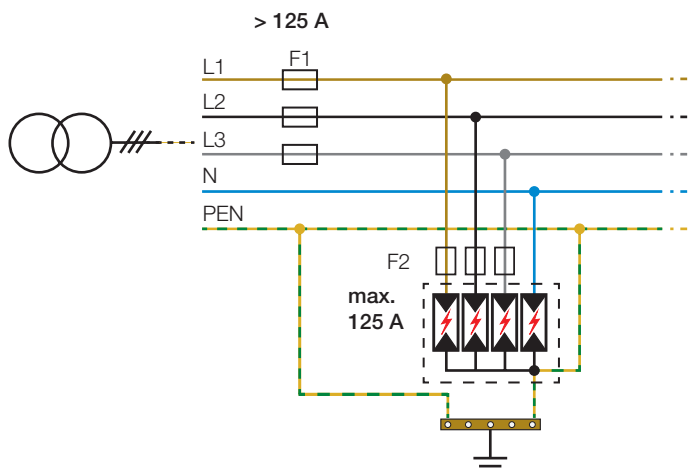
Abbildung 13: Notwendige Vorsicherung als Backup-Schutz für Überspannungsableiter
