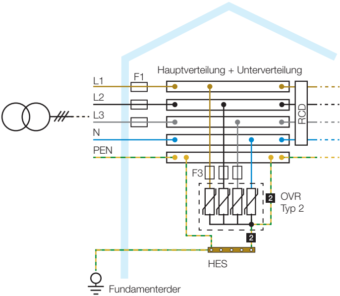
Abbildung 7: Einsatz von Überspannungsableitern in einem Wohngebäude ohne äußere Blitzschutzanlage und mit einem TN-S-System
