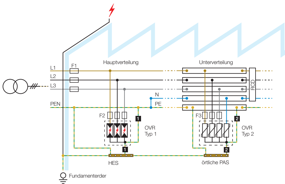
Abbildung 2: Einsatz von Blitzstrom- und Überspannungsableitern in einem Industriegebäude mit einem TN-C-S-System
