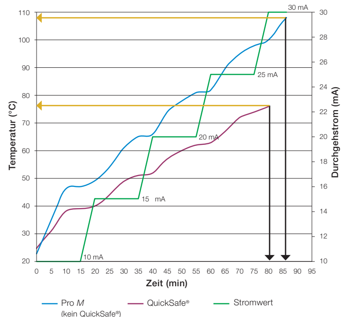
Thermische Abschaltung – am Abschaltpunkt des Metalloxidvaristors gemessene Temperaturen
