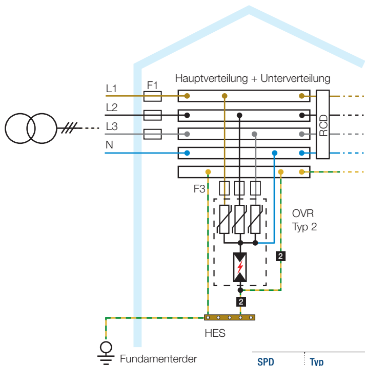
Abbildung 9: Einsatz von Überspannungsableitern in einem Wohngebäude ohne äußere Blitzschutzanlage und mit einem TT-System
