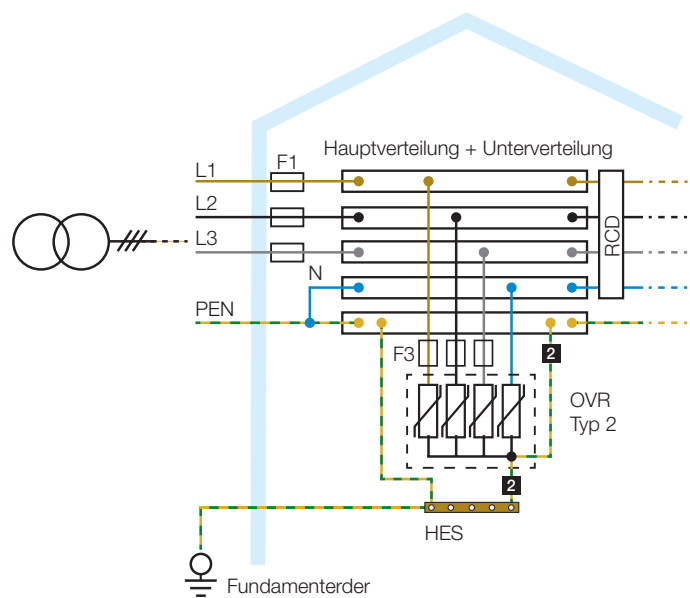
Abbildung 8: Einsatz von Überspannungsableitern in einem Wohngebäude ohne äußere Blitzschutzanlage und mit einem TN-C-S-System
