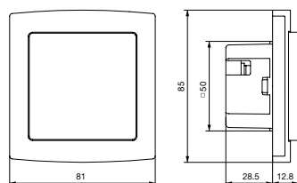
Maßzeichnung
