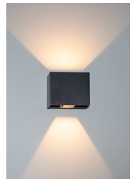
Abstrahlwinkel oben: 90° Abstrahlwinkel unten: 60°
