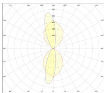
Asymmetrische Speziallinse 29° x 77° x 8°
