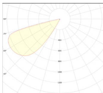
Lichtverteilungskurve von GUIDEround
