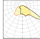
Lichtverteilung ASYM 50° x 110°
