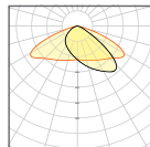
Lichtverteilung A SYM45° x 140°
