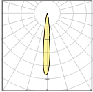
Lichtverteilung SYM 10
