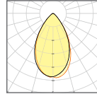
Lichtverteilung SYM 60
