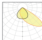
Lichtverteilung ASYM 48° x 92°
