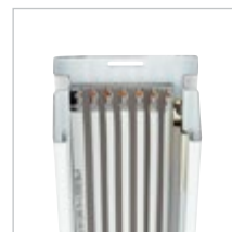
7-polig: 4 x 2,5 mm² + 2 x 1,5 mm² + PE
