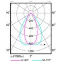
NB-HRO (tiefstrahlend-Hochregallageroptik)
