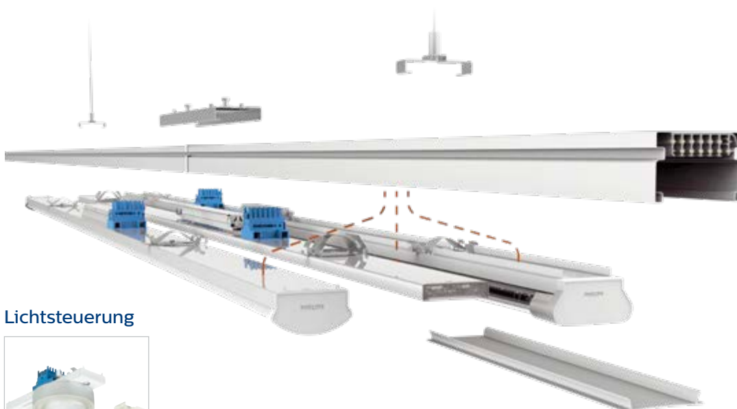
CPE: Außenkupplung (nur bei abgependelter Montage)
