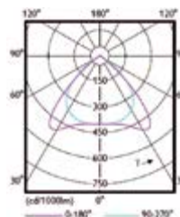
Breitstrahlend (WB)
