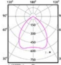
Breitstrahlend (WB) + Aluminiumreflektor
