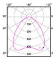
Breitstrahlend (WB)
