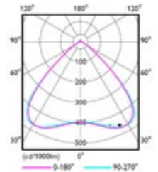
WB (breitstrahlend)
