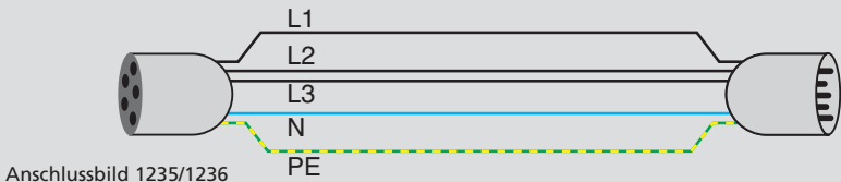
Anschlussbild 1235/1236
