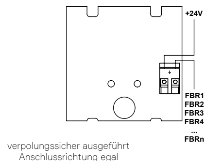
Verdrahtungsbeispiel:
