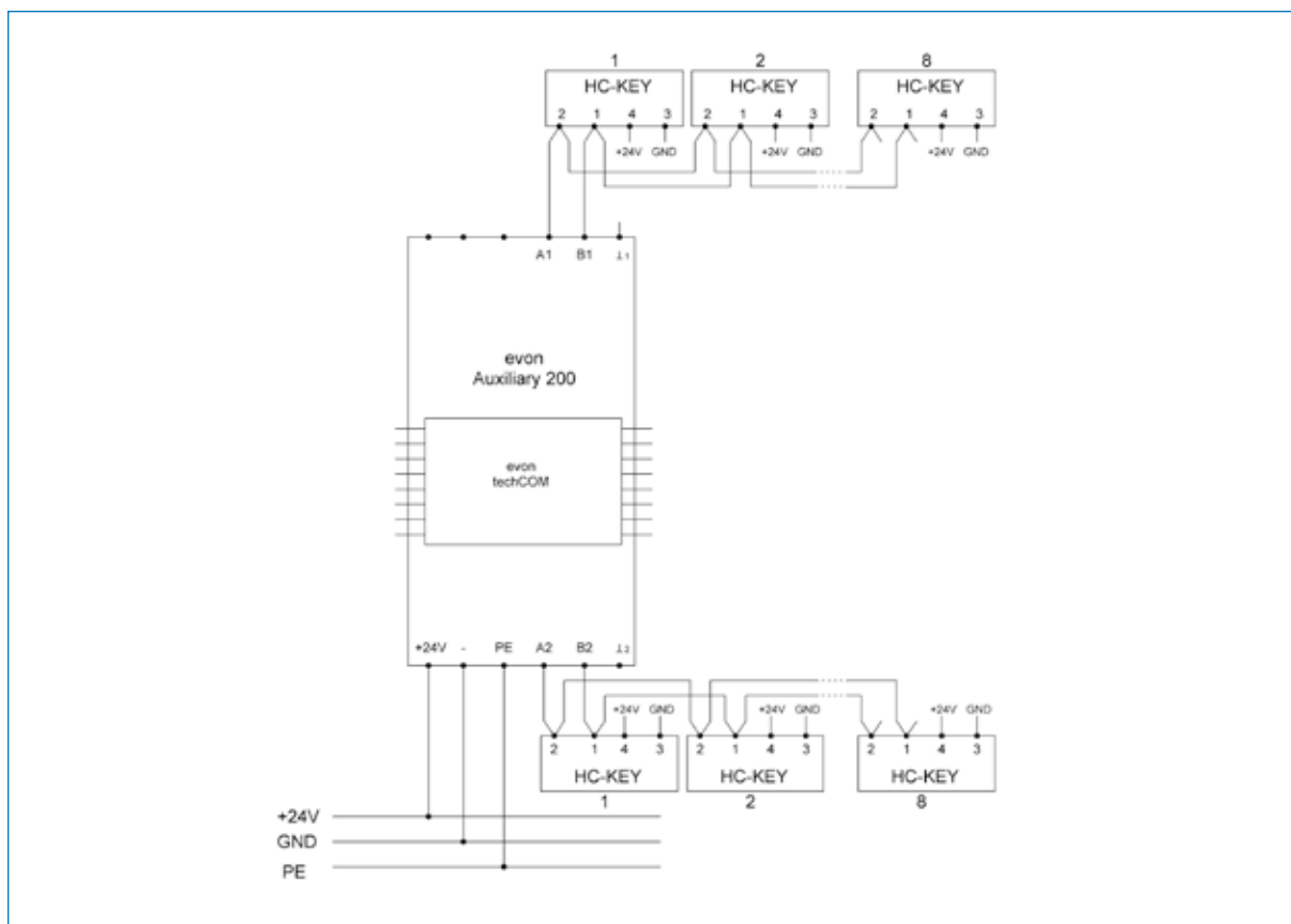
Verdrahtungsbeispiel KEYAP-00, KEYUPE-00, HC-KEYUPI-00
