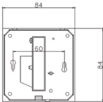
Befestigung / Montage:
