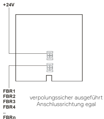
Verdrahtungsbeispiel:
