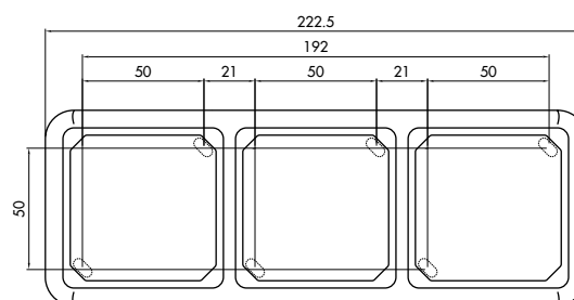
Aufputzgehäuse 3-fach
