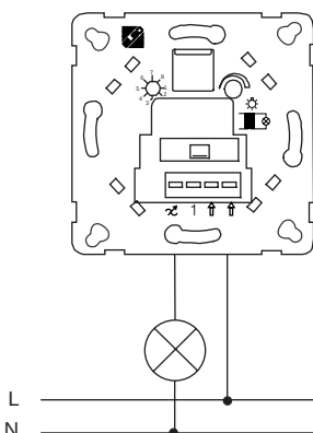
Triacgerät mit ohmscher Last, Art.Nr.: 171060
