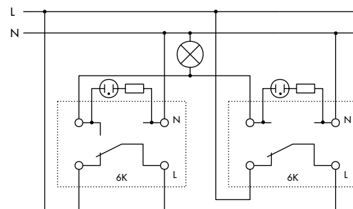
Kontroll-Wechselschaltung
