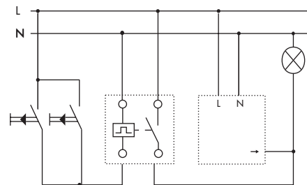
Bewegungsmelder mit Treppenhausautomatik
