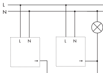
Parallelbetrieb mehrerer Bewegungsmelder auf einen Verbraucher
