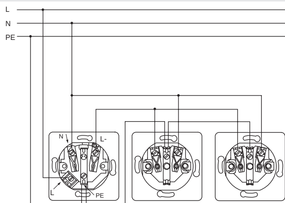
Schaltbild 2,5 kA
