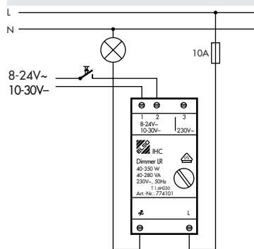
Steuerungsart 2, LR 350
