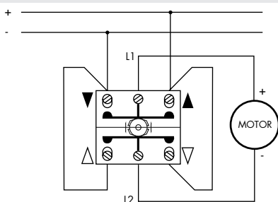
Jalousiedreheschalter, Pol-Wende-Schaltung
