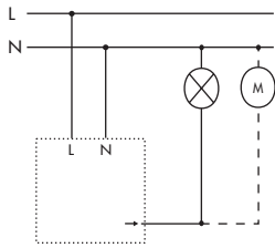
Durch zusätzliche Taster (Öffner) kann das Licht manuell von mehreren Stellen für eingestellte Zeit eingeschaltet werden
