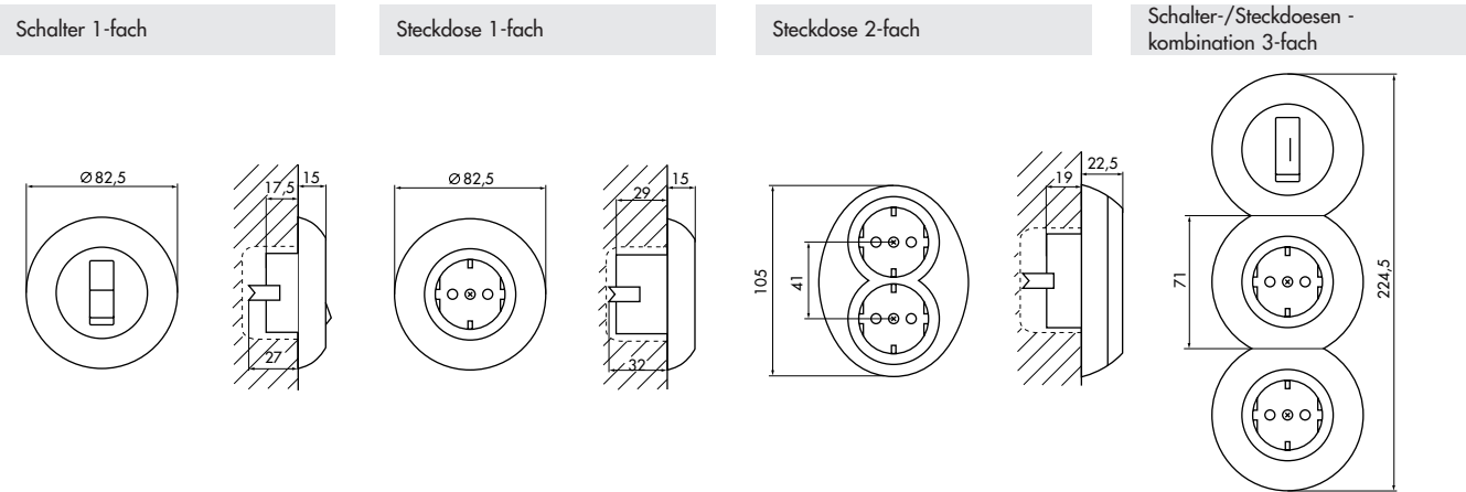
Rahmenabmessungen
