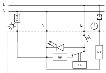
Temperaturregler als Öffner, Art. Nr.: 176241
