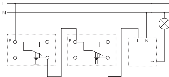
Durch zusätzliche Taster (Öffner) kann das Licht manuell von mehreren Stellen für eingestellte Zeit eingeschaltet werden
