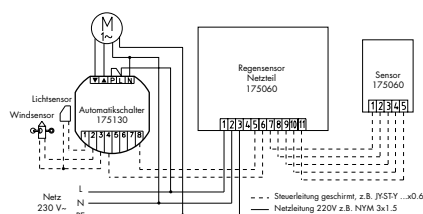
Regensensor, Art. Nr.: 175060
