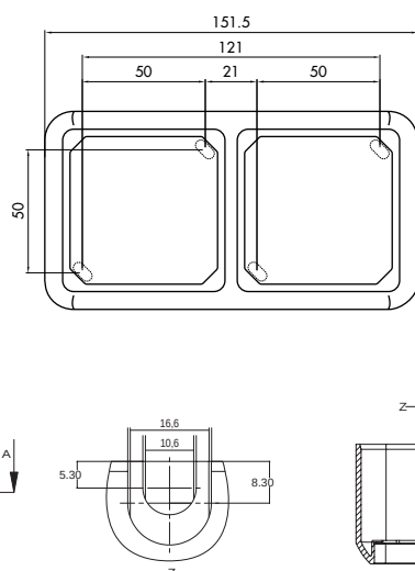
Aufputzgehäuse 2-fach
