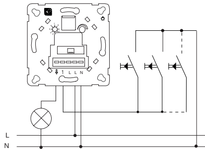
Nebenstellenschaltung, Art.Nr.: 171070
