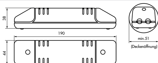
Transformatoren 60 W und 105 W
