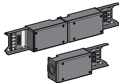
Einspeisung
