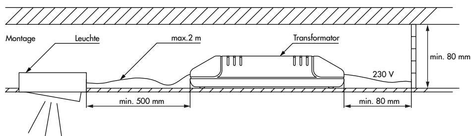
Montage in einer Zwischendecke
