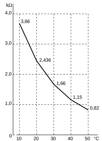
Kennlinie Fernfühler, Art. Nr.: 176130 u. 176150
