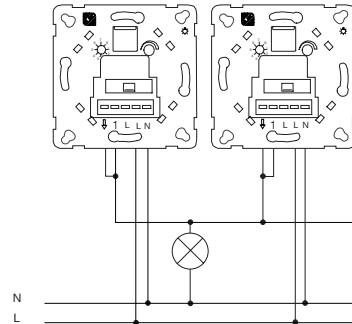
Anschlussbeispiel für Parallelbetrieb, Art.Nr.: 171070
