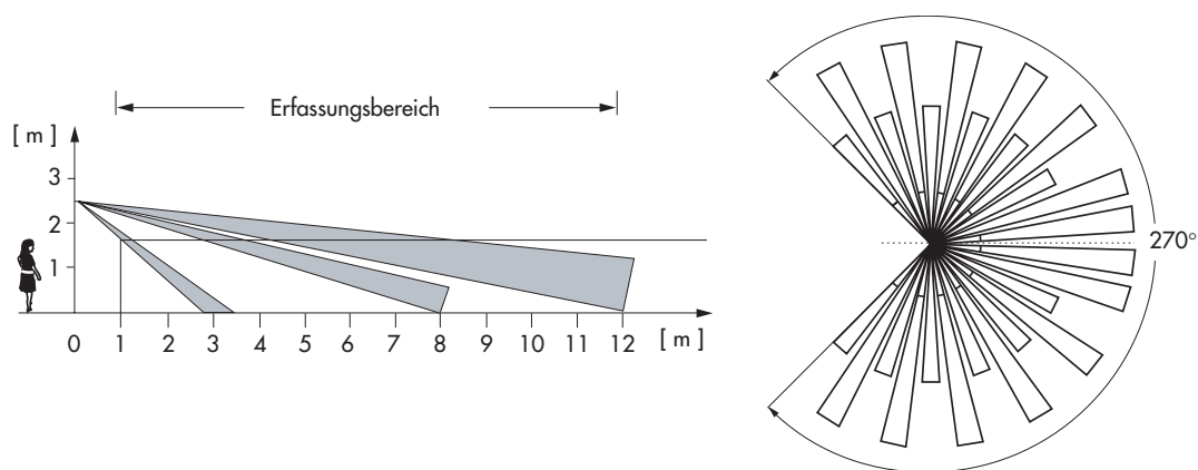
Aufbau Bewegungsmelder 270°
