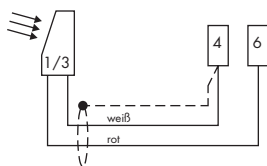
Anschluss eines zweiten Lichtaufnehmers
