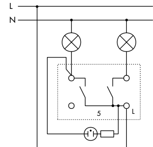
Serienschaltung / beleuchtet mit entsprechender Leuchtmarkierungsbaugruppe
