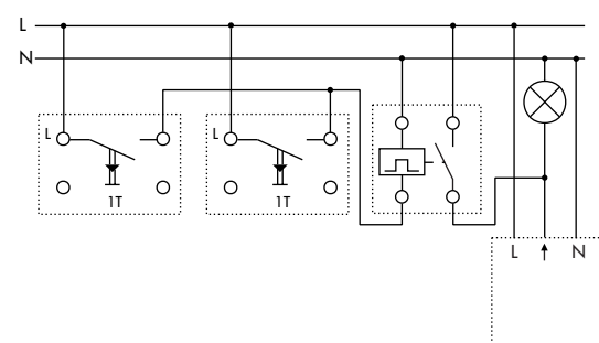
Parallelbetrieb Treppenhausautomat und Bewegungsmelder
