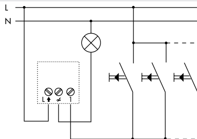
Nebenstellenschaltung mit Sensor- oder Tastdimmer
