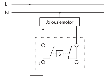
Jalousietaster, elektrisch und mechanisch verriegelt
