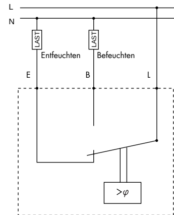
Schaltplan Hygrostat, Art. Nr.: 176301
