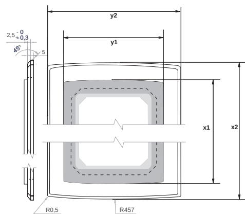
Rahmenabmessungen
