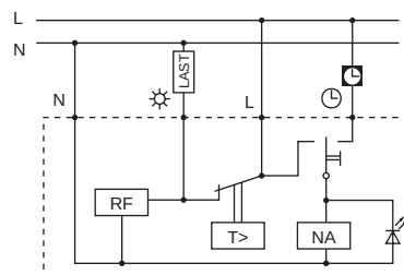
Schaltung als Öffner mit Wahlschalter, Art. Nr.: 176231
