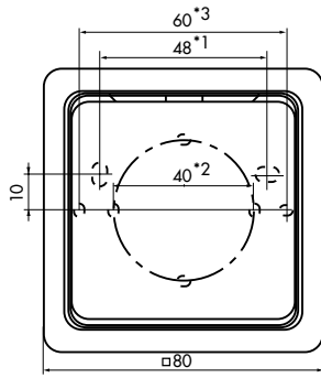
Befestigungsmaße
