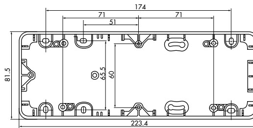
Aufputzgehäuse 3-fach
