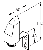
Lichtaufnehmer, Art. Nr.: 175040
