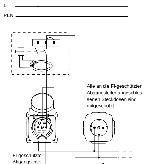
Anschlussbild TN-C-Netz
