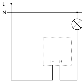
Bewegungsmelder am Netz
