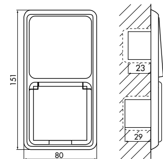
Schalter-/Steckdosenkombination
