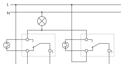
Sparwechselschaltung, beleuchtet
