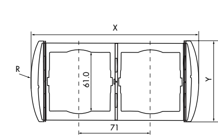
Rahmenabmessungen
