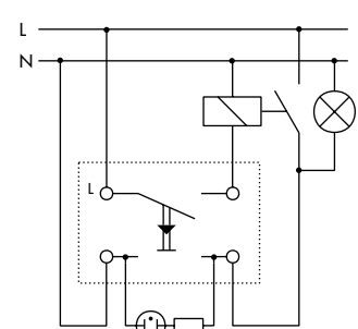
für Leuchtmarkierung mit Rückmeldung
