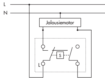
Jalousieschalter, elektrisch und mechanisch verriegelt
