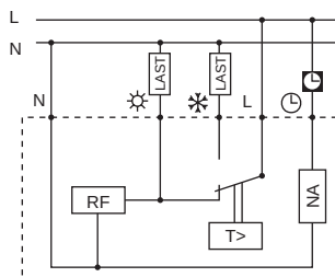
Schaltung als Wechsler, Art. Nr.: 176221
