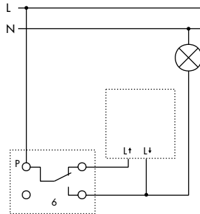
Umschaltung von Bewegungsmelder auf Dauerlicht
