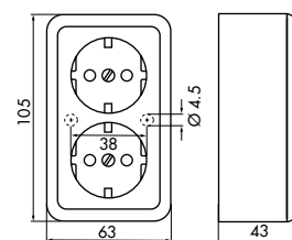
Steckdose 2-fach 2)
