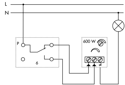
Ausschaltung mit Sensor- oder Tastdimmer
