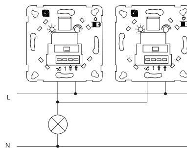
Anschlussbeispiel für Parallelbetrieb, Art.Nr.: 171060
