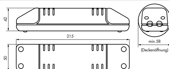
Transformatoren 150 W und 200 W
