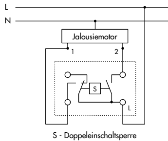
Jalousiedrehswitcher / Schlüsselschalter 2-polig
