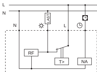
Schaltung als Wechsler, Art. Nr.: 176221
