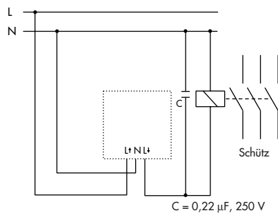
Parallelbetrieb Treppenhausautomat und Bewegungsmelder
