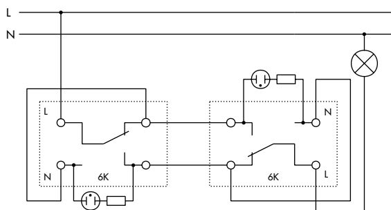
Kontroll-Wechselschaltung beleuchtet
