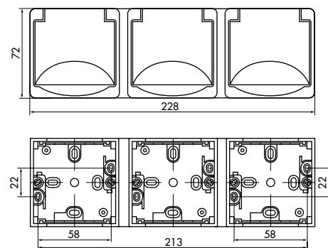
Steckdose 3-fach waagerecht
