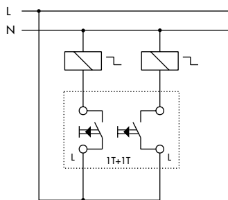
Doppeltaster (Zweifachtaster) mit getrennten Strombahnen
