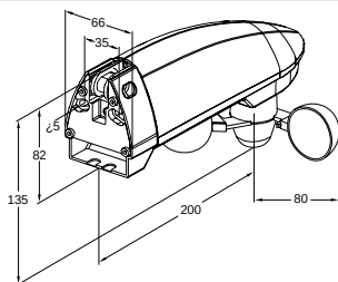
Licht-/ Windwächterkombination, Art. Nr.: 175051
