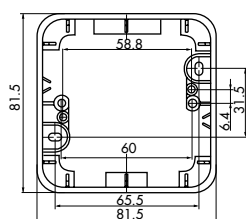
Aufputzgehäuse 1-fach
