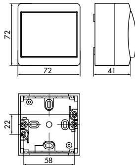
Schalter 1-fach
