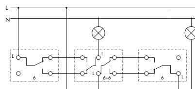
Wechselschaltung mit Doppelwechselschalter
