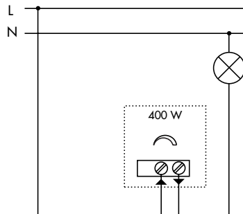
Ausschaltung mit Dimmer
