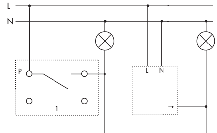
Bewegungsmelder mit Rückmeldung und Möglichkeit für Dauerlicht
