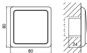
Schalter 1-fach
