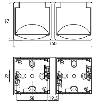
Steckdose 2-fach waagerecht
