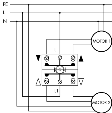
Jalousiedrehswitcher / Schlüsselschalter 2-polig
