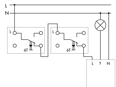
Bewegungsmelder mit Tastern (Öffner) - Nach Tastendruck schaltet der Melder f. d. vorgewählte Zeit ein, wenn er helligkeitsbedingt aktiv ist.
