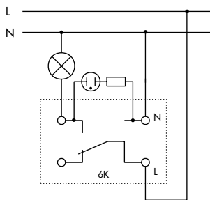
Kontroll-Ausschaltung, 1-polig
