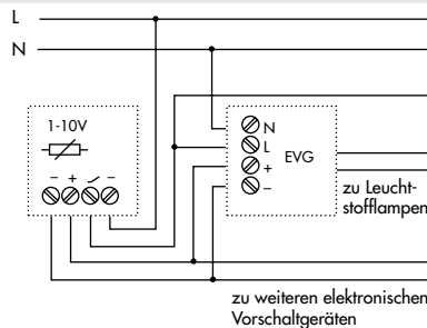
mit elektronischen Potentiometer
