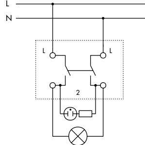
Kontroll-Ausschaltung, 2-polig
