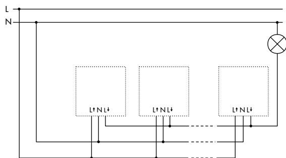
Parallelschaltung von Bewegungsmeldern
