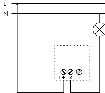
Ausschaltung mit Sensor- oder Tastdimmer
