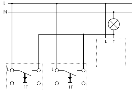
Bewegungsmelder mit Tastern - Nach Tastendruck schaltet der Bewegungsmelder für die vorgewählte Zeit ein, wenn er helligkeitsbedingt aktiv ist.
