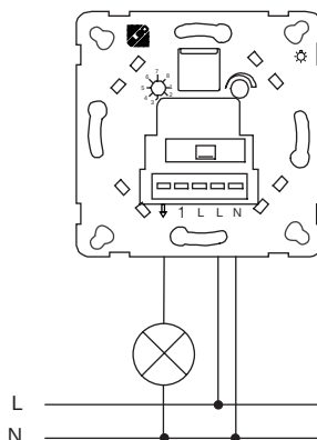
Relaisgerät mit ohmscher Last, Art.Nr.: 171070
