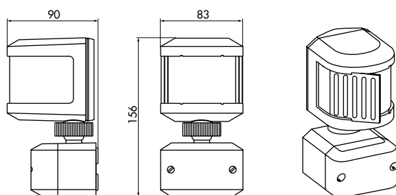
Aufbau Bewegungsmelder 270°
