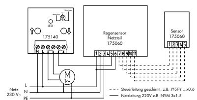
Regensensor, Art. Nr.: 175060
