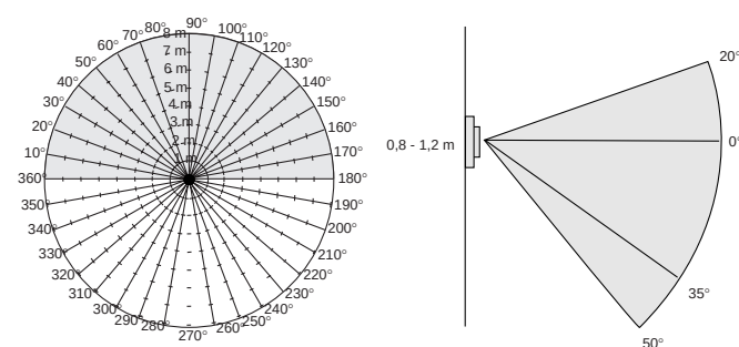
Erfassungsdiagramm Sensoraufsatz, Art.Nr.: 21706..., 29706...
