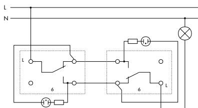
Wechselschaltung
