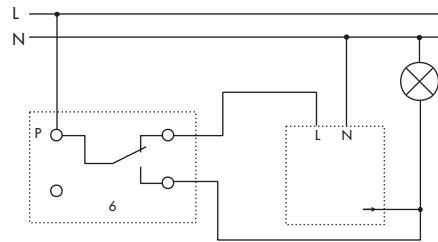
Umschaltung von Bewegungsmelder auf Dauerlicht
