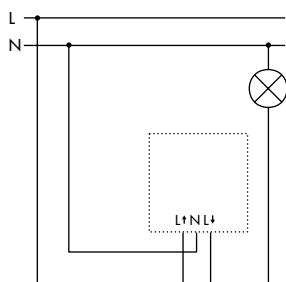
Parallelschaltung von Bewegungsmeldern
