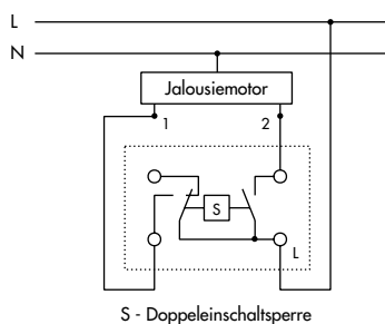
Jalousiedreheschalter, Pol-Wende-Schaltung
