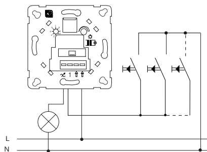
Nebenstellenschaltung, Art.Nr.: 171060
