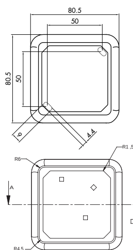
Aufputzgehäuse 1-fach
