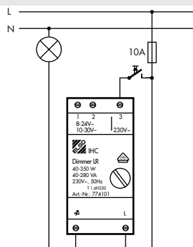
Steuerungsart 1, LR 350
