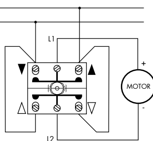
Jalousiedrehswitcher, Pol-Wende-Schaltung
