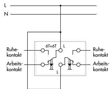
Doppelwechseltaster
