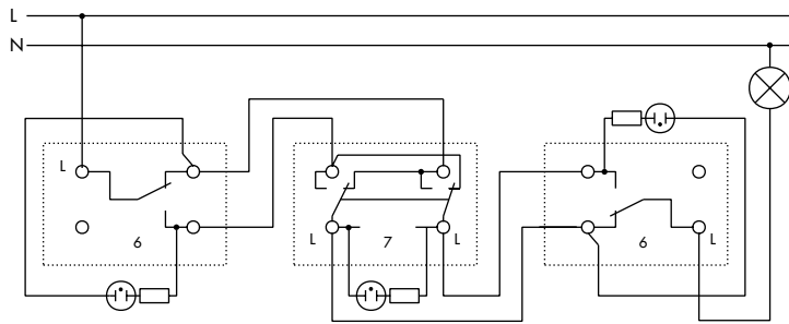
Kreuzschaltung / beleuchtet mit entsprechender Leuchtmarkierungsbaugruppe
