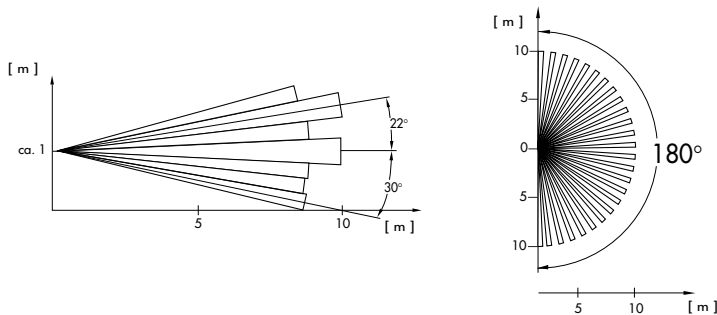
Erfassungsdiagramm Sensoraufsatz, Art.Nr.: 21706..., 29706...
