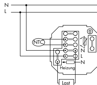
Temperaturregler mit Uhr 176140 (NTC Fühler entfällt) / 176150
