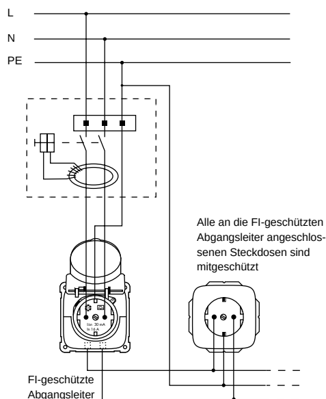
Anschlussbild TN-S- bzw. TT-Netz
