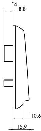
Unterputzmontage
