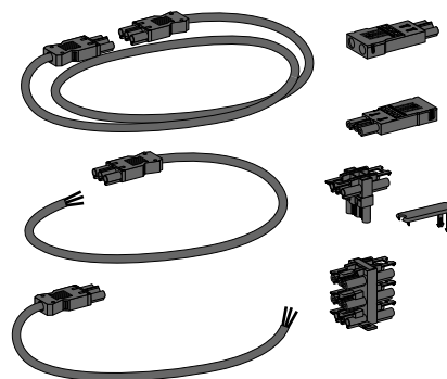
Vorgefertigte Anschlusstechnik
