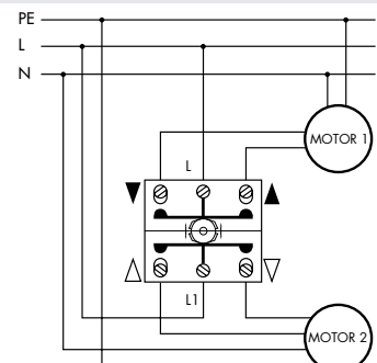
Jalousiedreheschalter / Schlüsselschalter 2-polig
