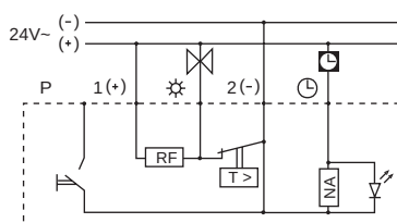
Temperaturregler als Öffner, Art. Nr.: 176241
