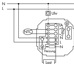
Temperaturregler 176160 (NTC Fühler entfällt) / 176130
