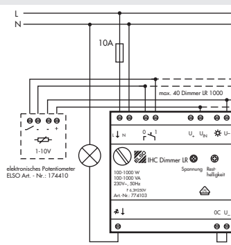
Steuerungsart 1, LR 1000
