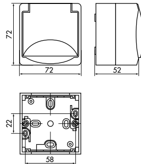
Steckdose 1-fach
