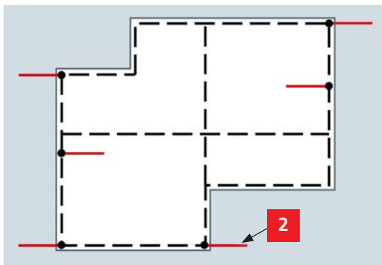
Erdungsfestpunkt Art.-Nr. 478 200
