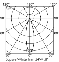
24w 3K 22°
