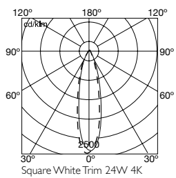
24w 4K 26°
