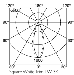
1w 3K 38°
