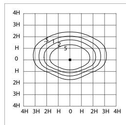
A2 Mini LED 43W H = 4.5m
