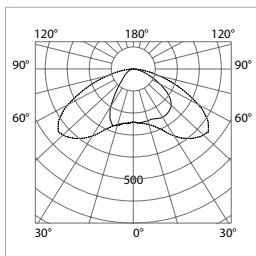
A2 Mini LED 43W — C0 - C180 - - - C90 - C270
