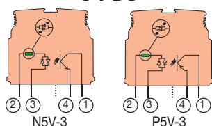
100 mA output optocoupler 5 V DC
