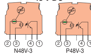
100 mA output optocoupler 48 V DC
