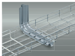
Eletrocalha aramada Cablofil, sete soluções para todos os ambientes.
