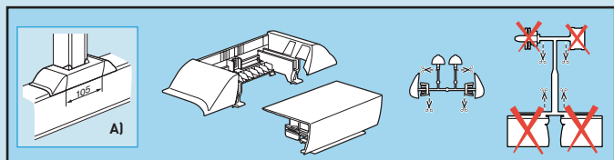
A) Exemplo de derivação em T utilizando uma derivação plana que possibilita a organização dos cabos com separadores internos.
