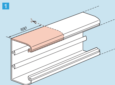
B) Utilizando a mesma derivação é possível fazer cotovelos 90 graus aproveitando os separadores internos com excelente acabamento
