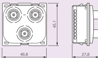
Tomada RCA 6630 84
