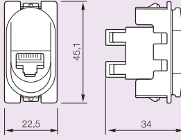
Tomada RJ45 Conexão 110 6630 79 / 6630 80
