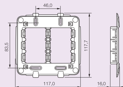
Suporte 4" x 4" 6121 24
