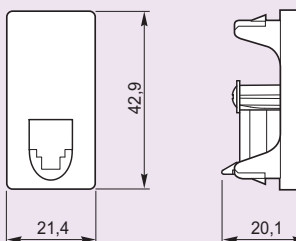
Tomada RJ 11 6150 11
