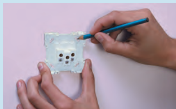
Definir o ponto, marcar, fazer a furação e fixar o mecanismo
