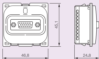
Tomada HD15 6630 83
