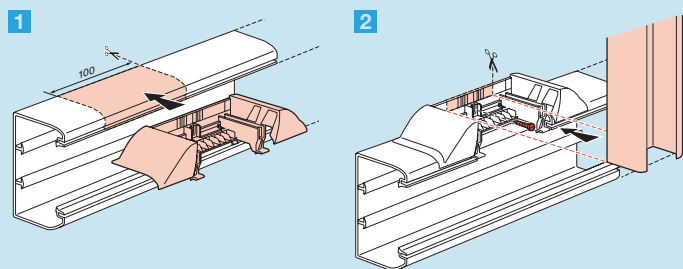
B) Utilizando a mesma derivação é possível fazer cotovelos 90 graus aproveitando os separadores internos com excelente acabamento
