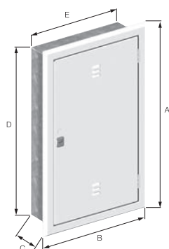
rack residencial embutir
