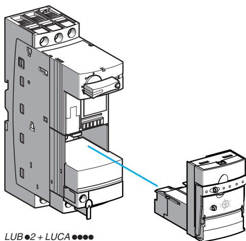
LUB●2 + LUCA●●●●
