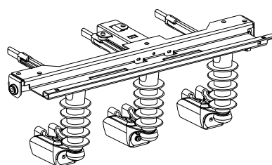
Chave terra 24 kV
