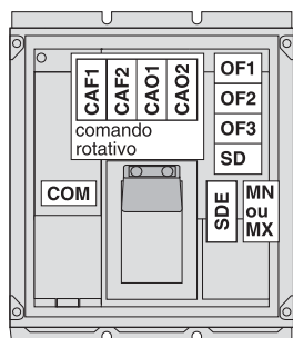
Dispositivo com comando manual
