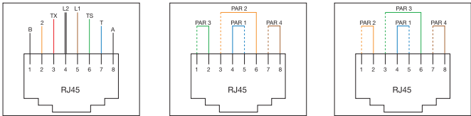
RJ45 (8 fios) Para linhas telefônicas
