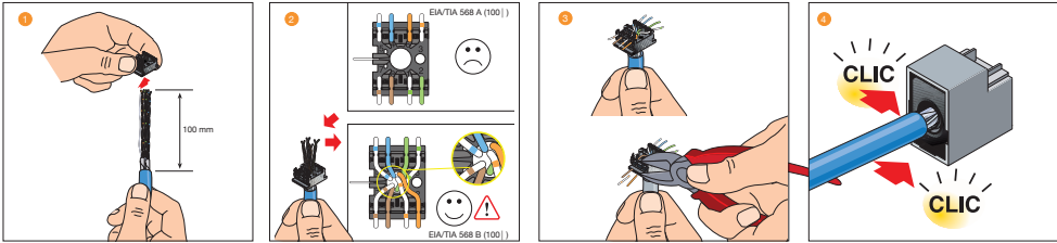
RJ45 (8 fios) Para linhas telefônicas
