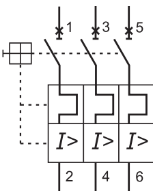
Esquema elétrico trifásico
