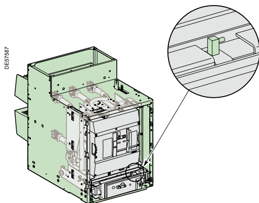
Interlocking door-cubicle
