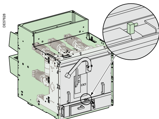
Interlocking door-cubicle
