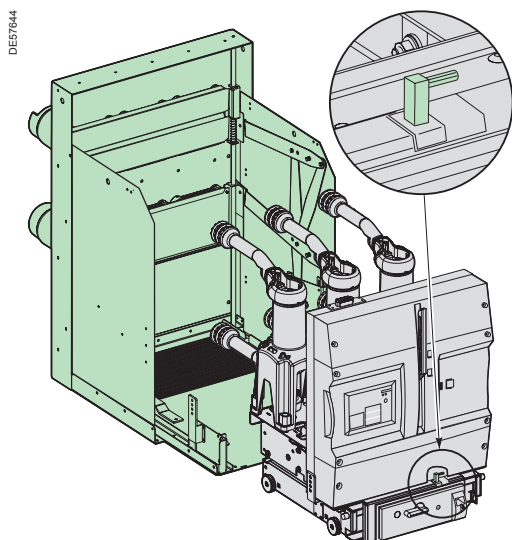
Interlocking door-cubicle
