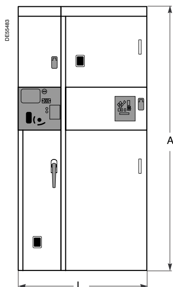
Vista frontal Cubículo principal soft starter
