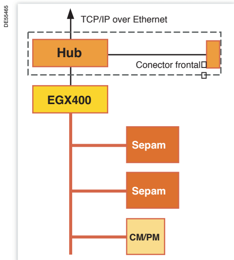
Centro de Controle de Motor Motorpact
