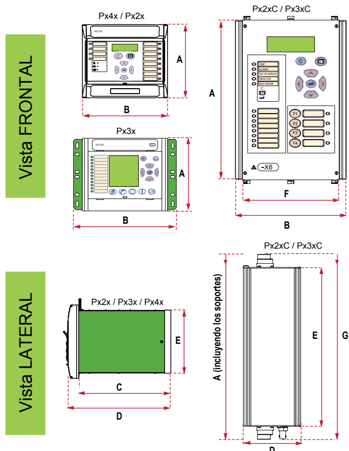
Figura 9 Dimensiones típicas de la caja
