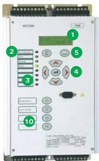
Figura 6: Interfaz de usuario diseño compacto
