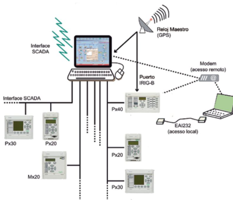
Figura 5 - Un sistema de control de subestación típico
