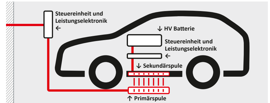
Abbildung 5: Prinzip induktives Laden
