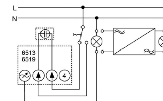
Wechselschaltung
