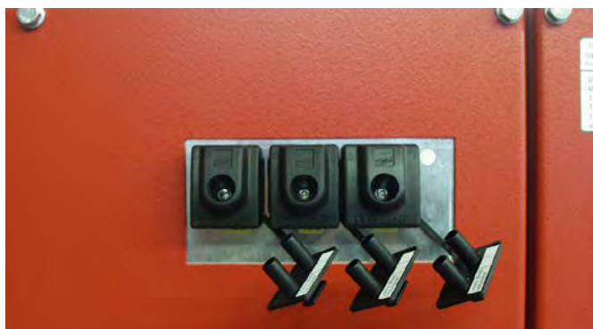
Passives Spannungsanzeigergerät DEHNcap/P an einer gekapselten Schaltanlage.
