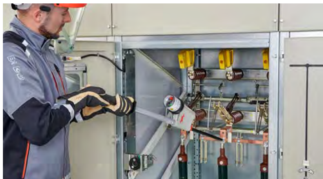
Spannungsprüfer PHE4 mit optischer und akustischer Anzeige.
