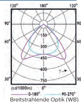
Breitstrahlende Optik (WB)
