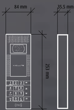
Módulo electrónico
