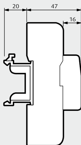
2 módulos
