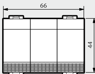
3 módulos
