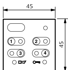
2 módulos AXOLUTE
