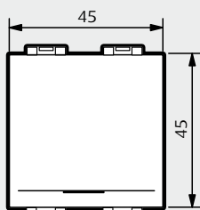
2 módulos
