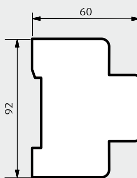
4-8-10 módulos
