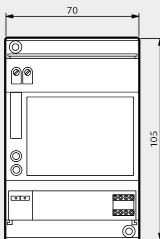
4 módulos
