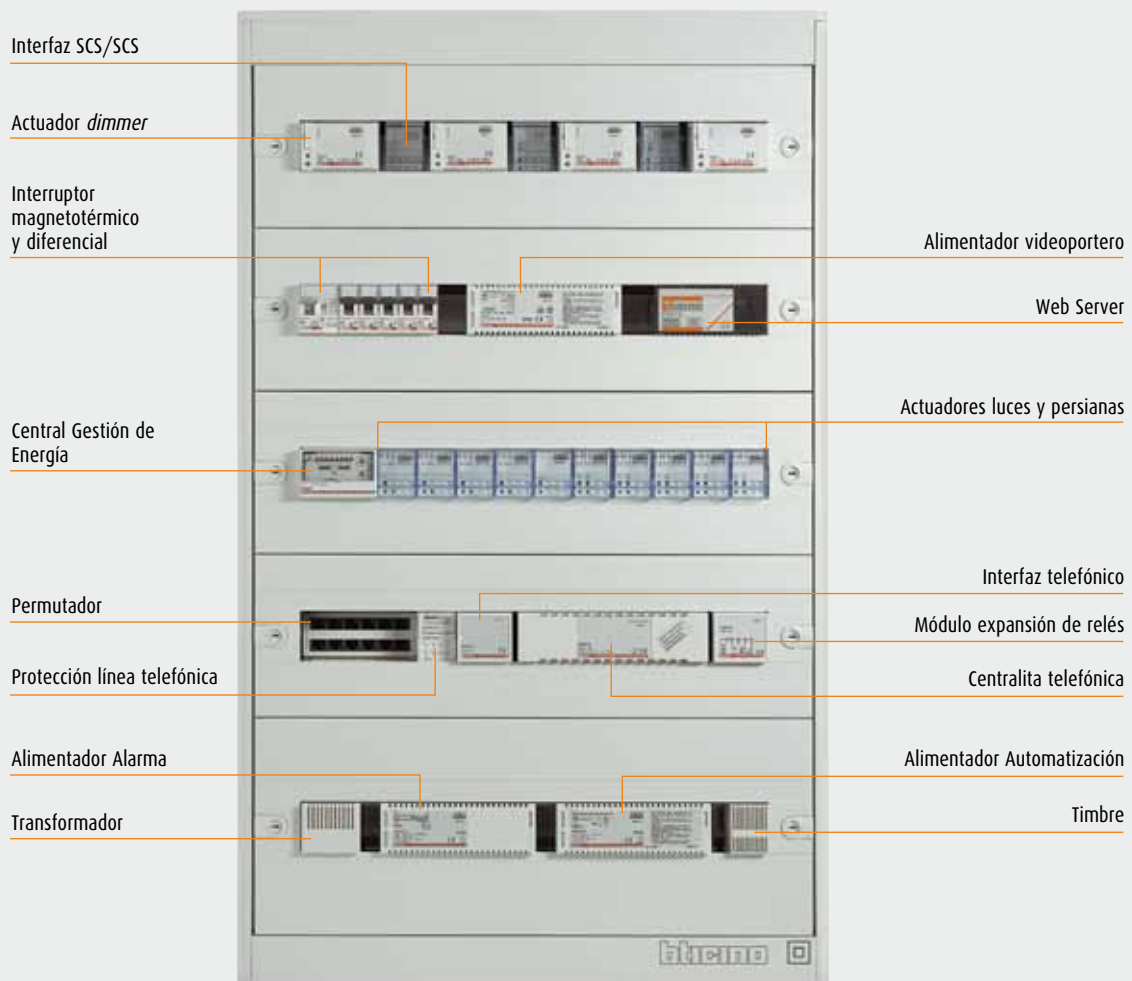
Ejemplo de una centralización domótica
