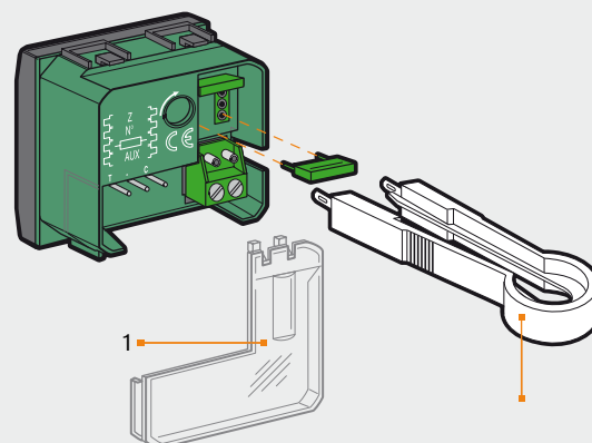
Insertión/extracción de los configuradores
