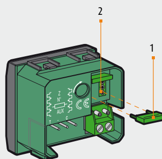
Alojamientos para la configuración de los dispositivos
