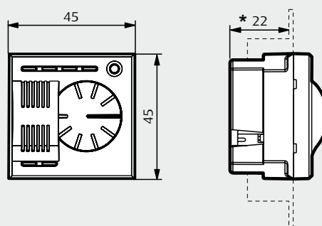
SONDA AXOLUTE
