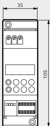
2 módulos
