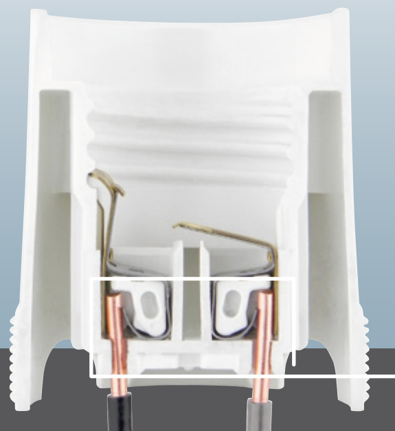
Bornes automáticos
