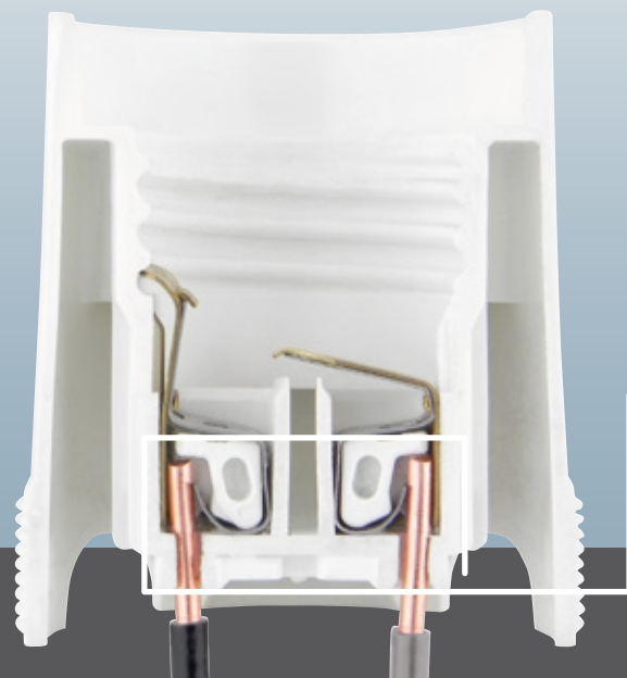
Bornes automáticos
