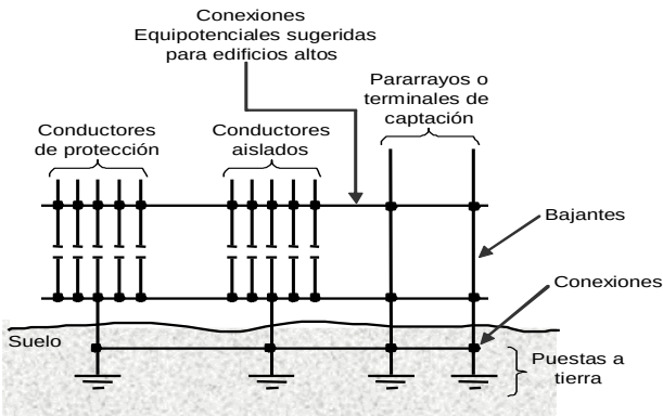
Figura 13.1.1 Sistemas con puestas a tierra dedicadas e interconectadas
