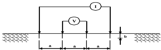
Figura 13.4.1.1. Esquema de medición de resistividad aparente
