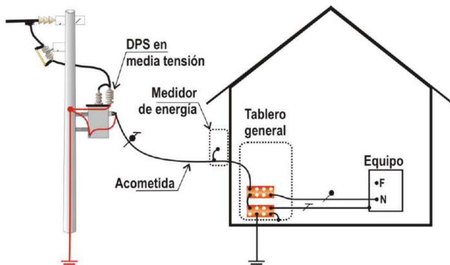
Figura 26.1 Esquema indicativo del régimen de conexión a tierra TN-C-S
