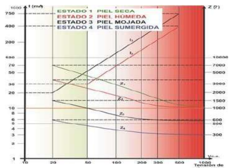
Figura 1.6.2. Impedancia del cuerpo humano
