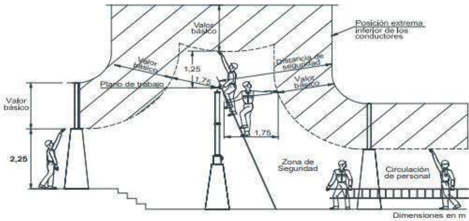
Figura 23.1.3 Zonas de seguridad
