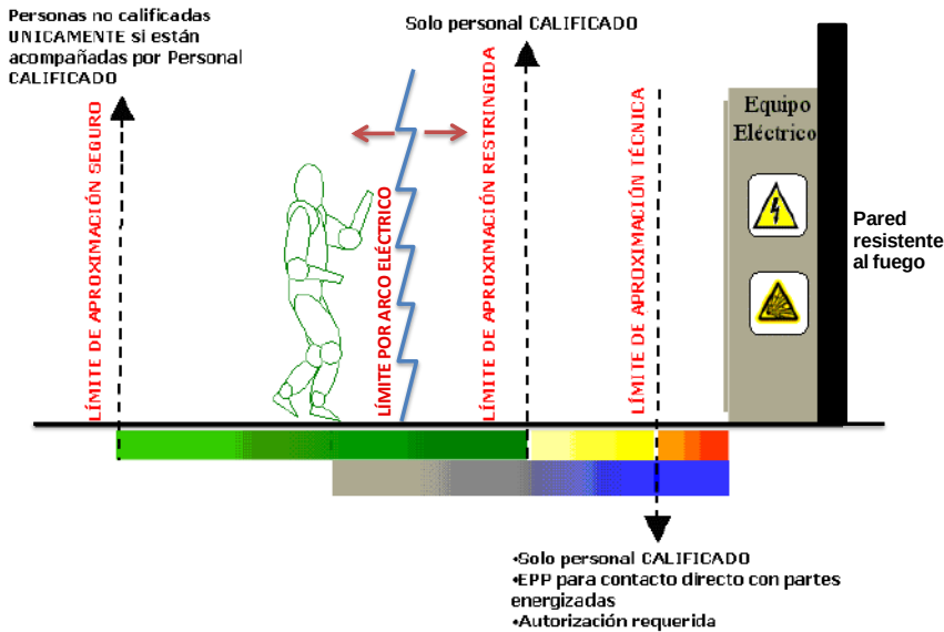
Figura 11.5.1. Límites de aproximación
