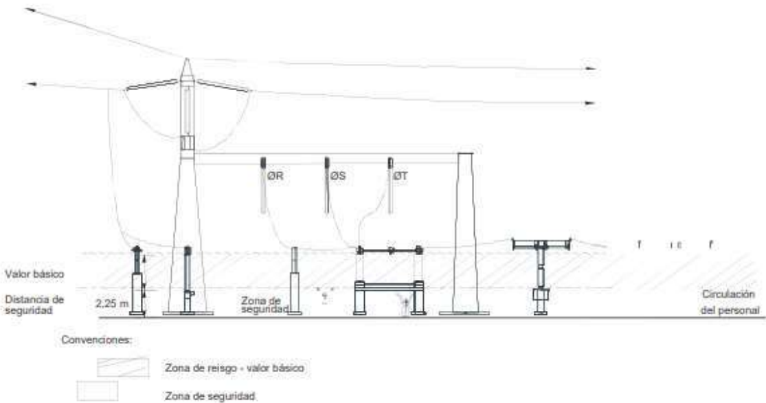
Figura 23.1.2 Zona de seguridad para circulación de personal
