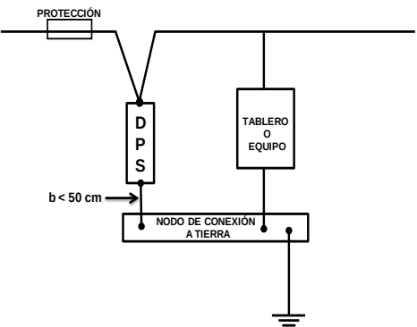
Figura 18.15.1. Montaje típico de DPS
