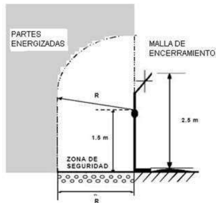
Figura 23.1.1 Distancias de seguridad para prevenir contactos directos en subestaciones exteriores
