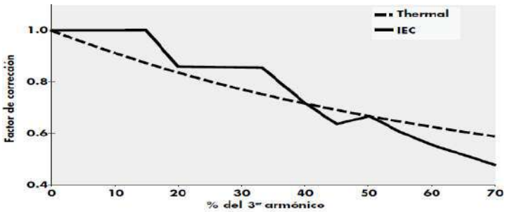
Figura 18.7.2.1 Factor de Corrección en función de la proporción de armónicos
