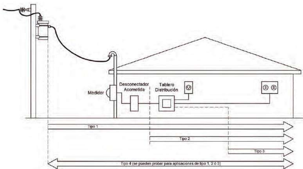
Figura 18.15.2. Ubicación de los DPS tipo 1, 2, 3 y 4
