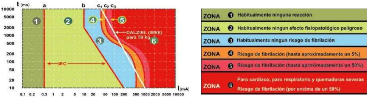
Figura 1.6.1 Zonas de tiempo/corriente de los efectos de las corrientes alternas de 15 Hz a 100 Hz
