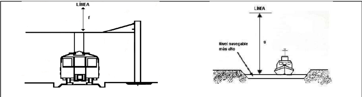
Figura 11.2.3. Distancia “f” y “g” para cruces con ferrocarriles y ríos
