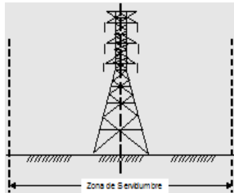
Figura 20.1.1 Ancho de la zona de servidumbre
