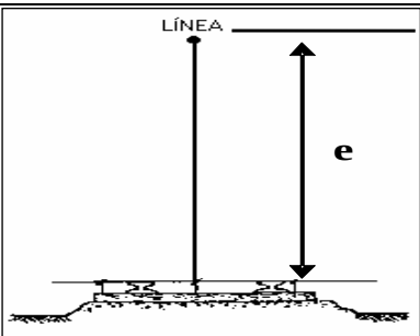
Figura 11.2.2. Distancia “e” en cruces con ferrocarriles sin electrificar
