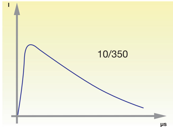
Protectores contra sobretensiones del Tipo 1 I_{imp} : Onda de corriente
