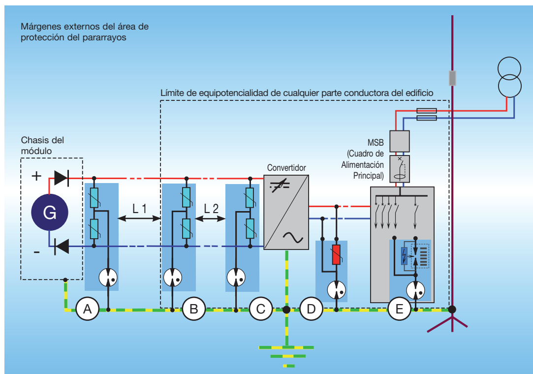
Ejemplo de diagrama de una instalación de 600 V
