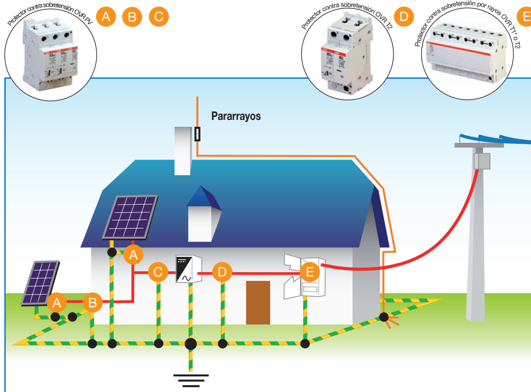
Ejemplo de instalación típica
