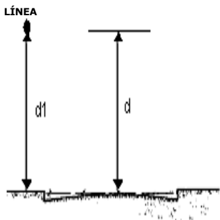
Figura 6. Distancias “d” y “d1” en cruce y recorridos de vías
