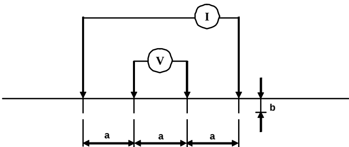
Figura 13. Esquema de medición de resistividad aparente.
