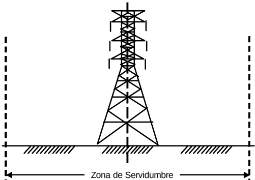
Figura 19. Ancho de la zona de servidumbre.
