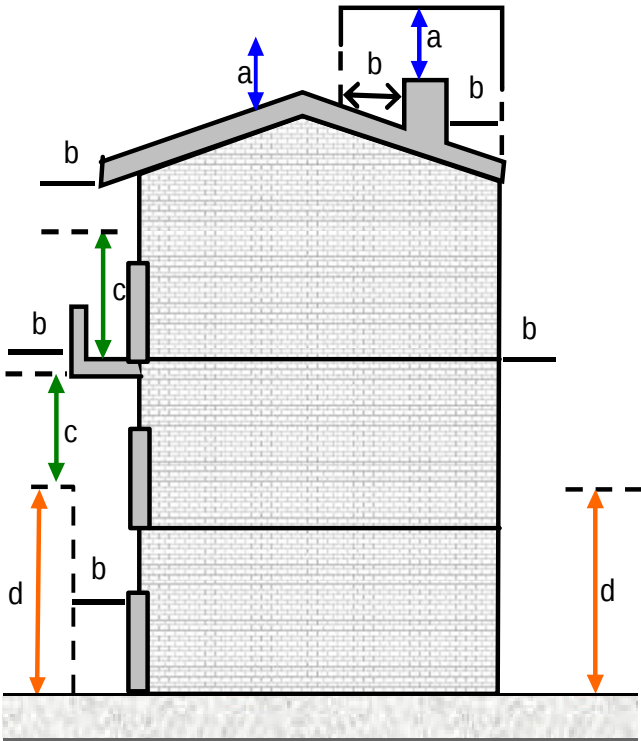
Figura 5. Distancias de seguridad en zonas con construcciones
