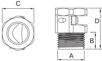
Abmessungen
