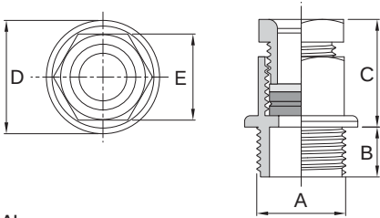
Abmessungen
