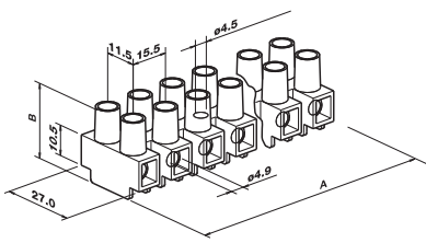
Abmessungen
