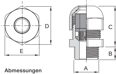
Abmessungen
