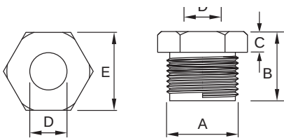
Abmessungen
