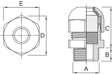
Abmessungen
