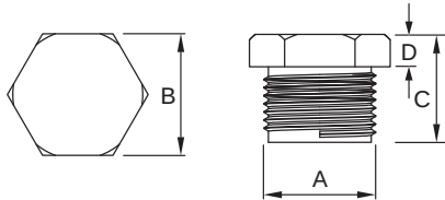
Abmessungen
