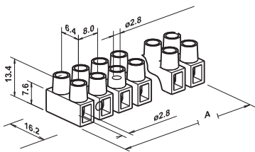
Abmessungen
