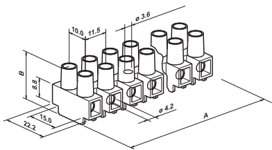
Abmessungen
