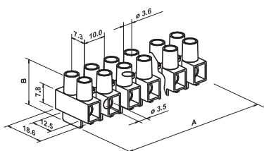
Abmessungen
