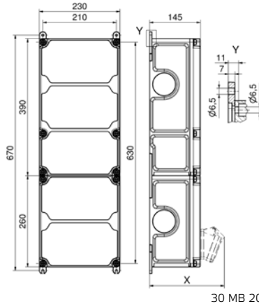
Tiefenmaß X (in mm)
