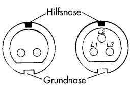
Steckdose Vorderseite
