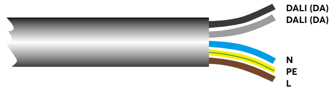
Abbildung: Typischer Aufbau der verwendeten Kabel
