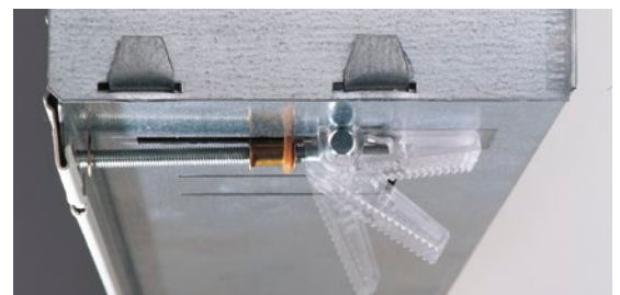
Hohlwandset ZKV200P4 einsetzen, fixieren, fertig
