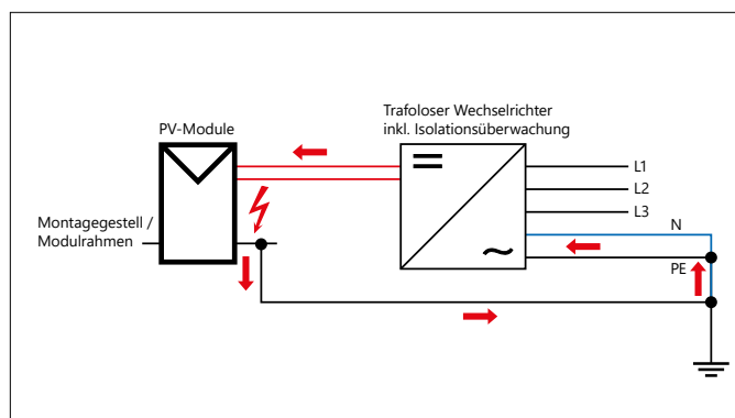
Isolationsfehler im DC-System bei trafolosen Wechselrichtern
