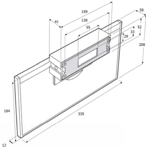
Primora 82 W Gehäuse oben (ZBL)
