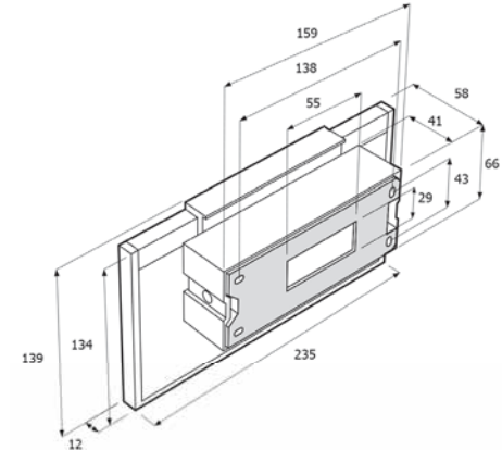
Primora 81 W Gehäuse oben (EBL)
