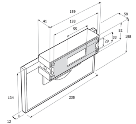
Primora 81 W Gehäuse oben (ZBL)
