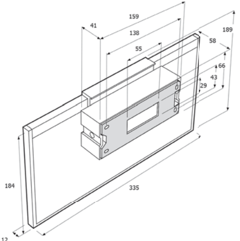
Primora 82 W Gehäuse oben (EBL)
