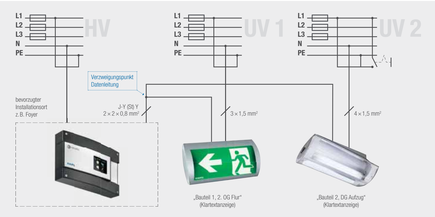
Installationsschema
