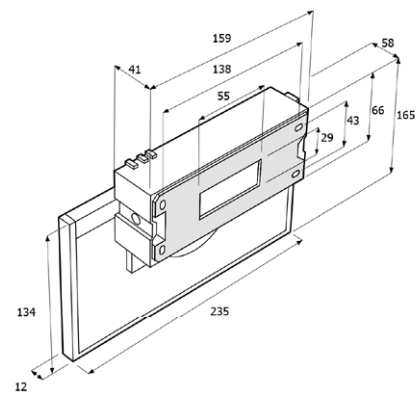
Primora 81 W Gehäuse oben (EBL)
