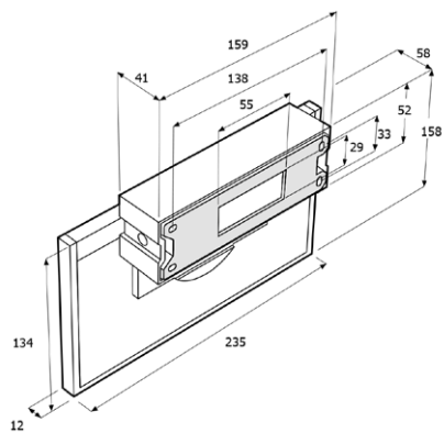
Primora 81 W Gehäuse oben (ZBL)
