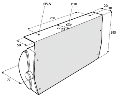
Aqualux 25 D (eins.)
