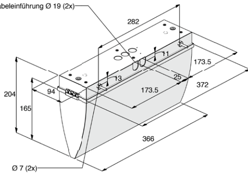
Optima 14L 32 m W
