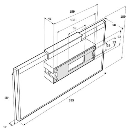
Primora 82 W (ZBL)
