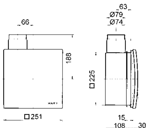
Ventilatoreinsatz ER mit Unterputzgehäuse ER-UP/G oder ER-UPD
