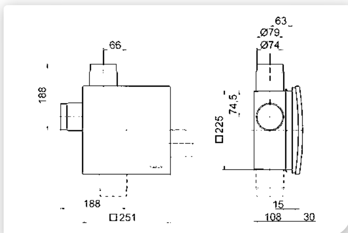
ER-UPD mit Zweitraumanschluss
