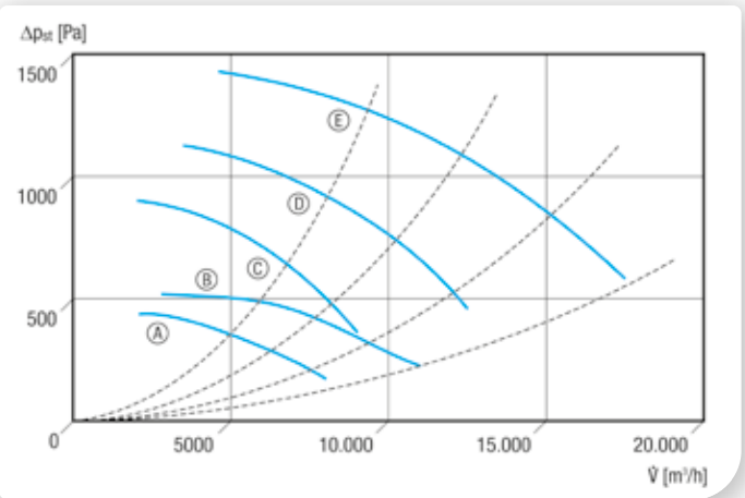
Kennlinien für Baugröße 500, 560 und 630, 4- und 6-polig
