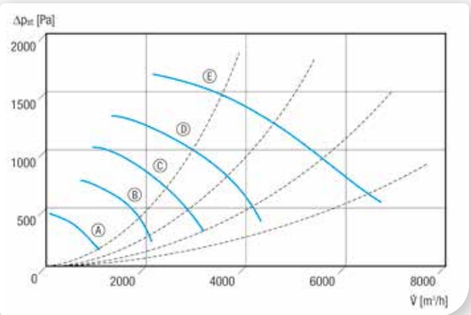
Kennlinien für Baugröße 200, 250, 280, 310 und 350, 2-polig
