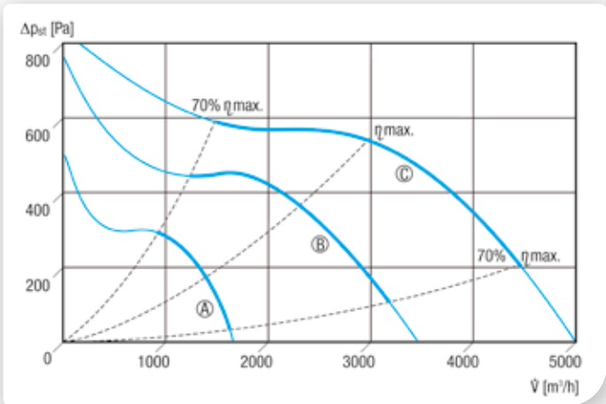
Ⓐ EDR 25 Ⓑ EDR 31 Ⓒ EDR 35
