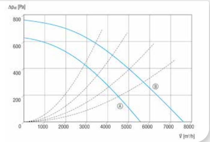
Ⓐ EKR 35-2 Ⓑ EKR 40-2
