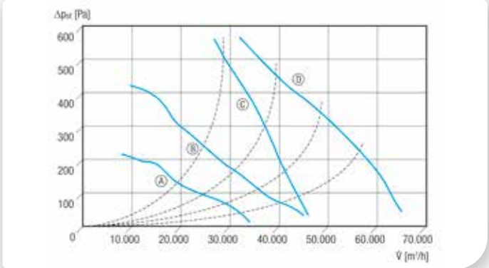
Ⓐ DAS 100/8 Ⓑ DAS 100/6 Ⓒ DAS 90/4 Ⓓ DAS 100/4
