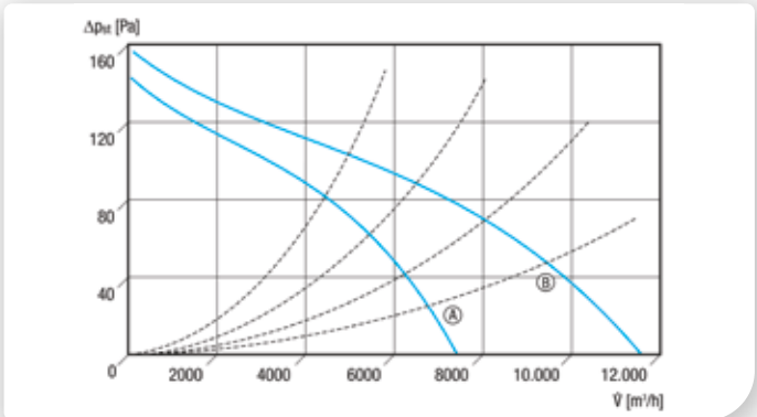
Ⓐ DAD 63/6 Ⓑ DAD 71/6
