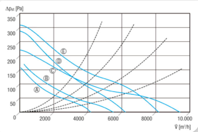
Kennlinien für DN 450 bis DN 600
