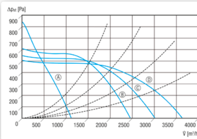
Ⓐ MDR 18 EC, MDR-PG 18 EC Ⓑ MDR 22 EC, MDR-PG 22 EC Ⓒ MDR 25 EC, MDR-VG 25 EC Ⓓ MDR 31 EC, MDR-VG 31 EC
