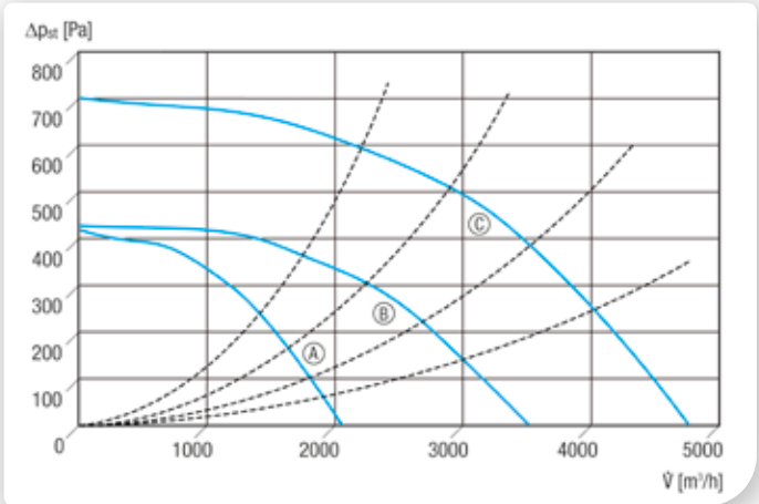
Ⓐ DSK 22 EC Ⓑ DSK 31 EC Ⓒ DSK 31/1-S EC
