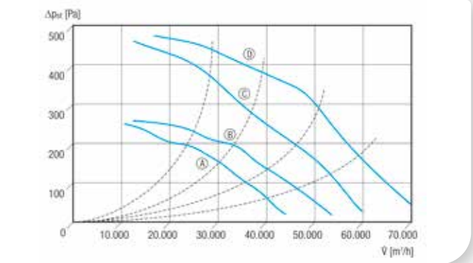
Ⓐ DAS 112/8 Ⓑ DAS 125/8 Ⓒ DAS 112/6 Ⓓ DAS 125/6
