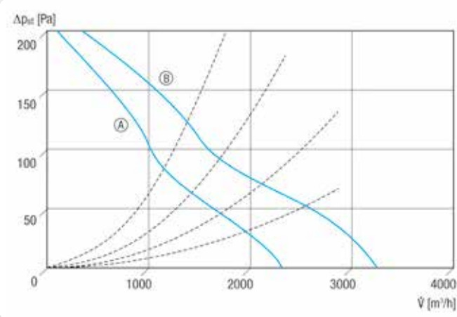
Ⓐ EZD, DZD 35/4 B Ⓑ EZD, DZD 40/4 B
