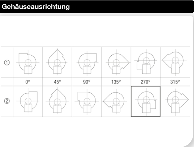
① Rechtsausführung ② Linksausführung
