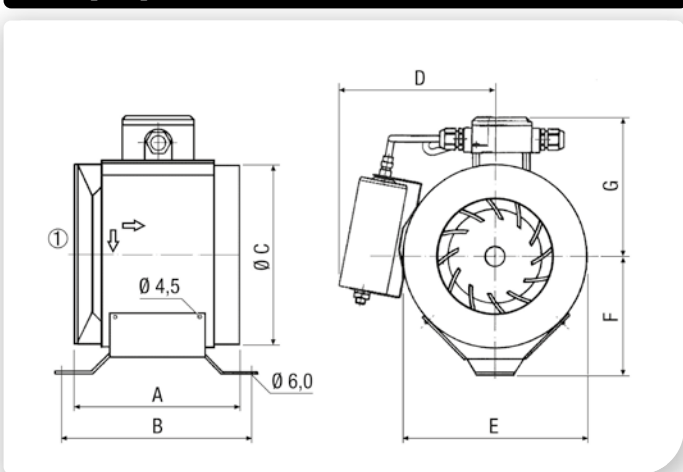
Ⓐ ERM 22 Ex t und ERM 22 Ex t/60 Hz: 2 Reduzierstücke auf DN 200 im Lieferumfang enthalten. Nicht in der Maßzeichnung abgebildet.
