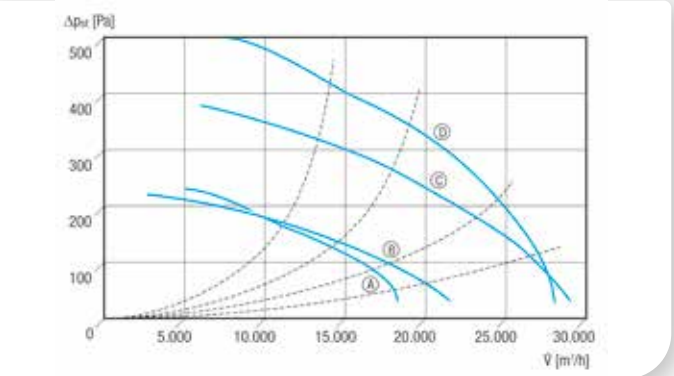
Ⓐ DAS 80/6 Ⓑ DAS 90/8 Ⓒ DAS 90/6 Ⓓ DAS 80/4
