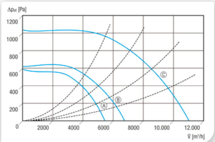
Ⓐ MDR 35 EC Ⓑ MDR 40 EC Ⓒ MDR 45 EC
