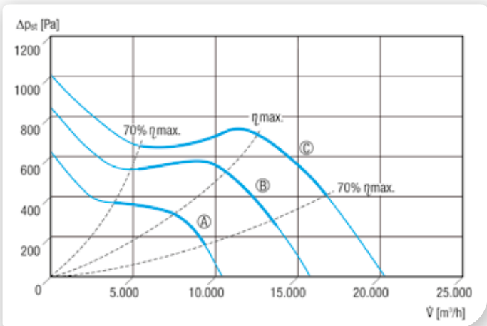
Ⓐ EDR 56 Ⓑ EDR 63 Ⓒ EDR 71
