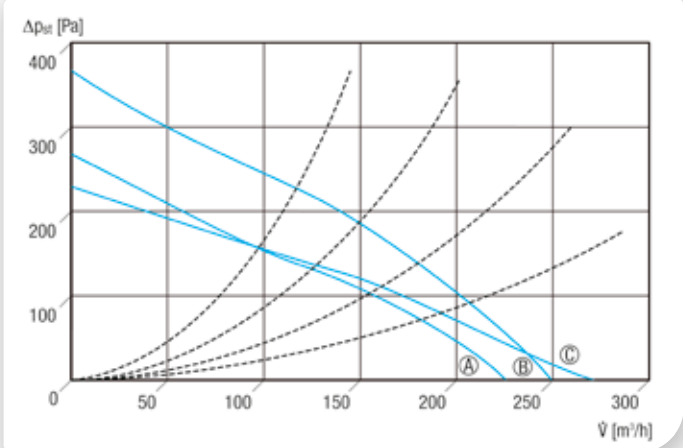
Ⓐ ERR 10/1 Ⓑ ERR 10/1 S Ⓒ ERR 12/1
