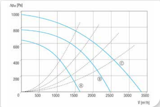
Ⓐ EKR 20-2 Ⓑ EKR 25-2 Ⓒ EKR 31-2
