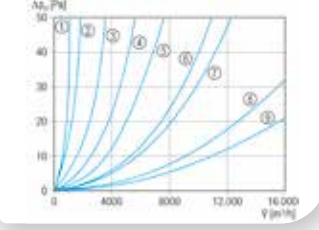
Druckverluste
