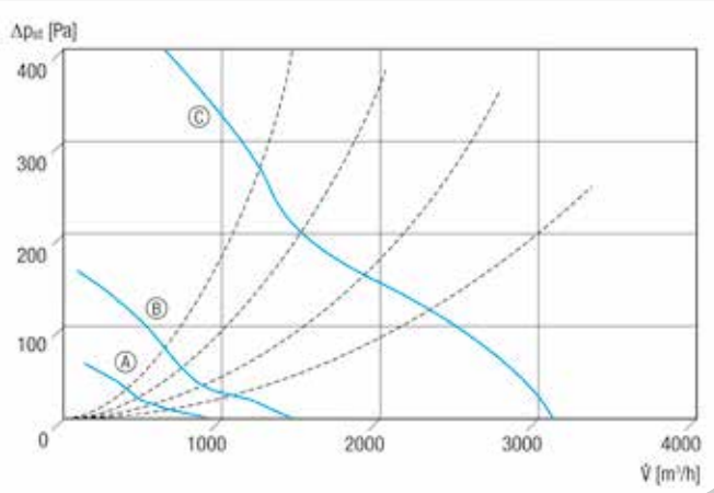
Ⓐ EZD 30/6 B Ⓑ EZD, DZD 30/4 B Ⓒ EZD, DZD 30/2 B
