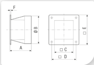
Maße [mm] URRI GR 16 bis URRI GR 35
