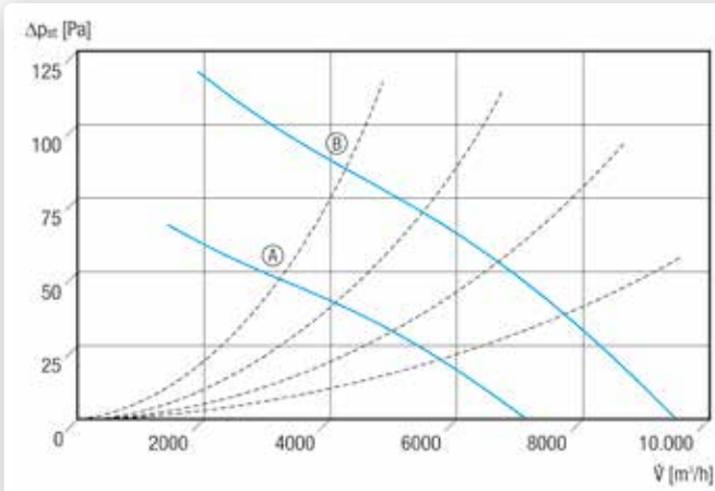
Ⓐ DAQ 63/8 Ex Ⓑ DAQ 63/6 Ex
