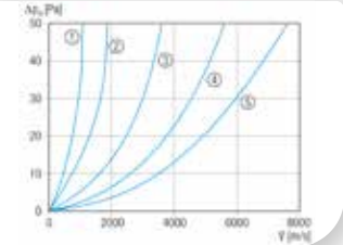
Druckverluste
