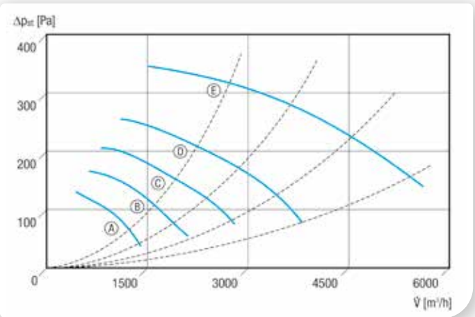
Kennlinien für Baugröße 310, 350, 400, 450 und 500, 6-polig
