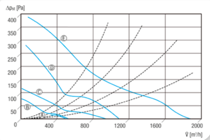
Kennlinien für DN 200 und DN 250
