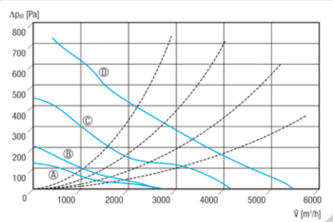
Kennlinien für DN 350 und DN 400
