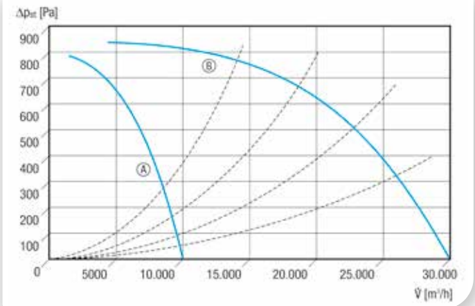
Ⓐ DRD H 50/4 Ⓑ DRD H 90/6
