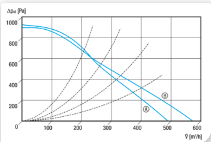
Ⓐ ESR 12-3 EC Ⓑ ESR 16-3 EC
