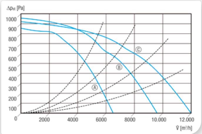
Ⓐ DSK 35/1 EC Ⓑ DSK 50 EC Ⓒ DSK 56 EC
