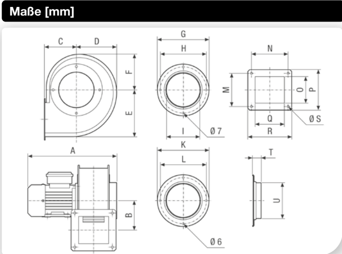
Maße G, H, I beziehen sich auf die Ansaugdüse, welche im Lieferumfang enthalten ist.
