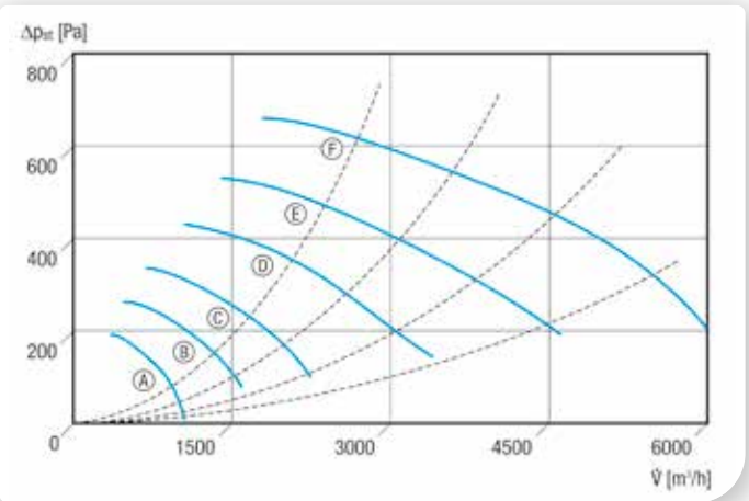
Kennlinien für Baugröße 250, 280, 310, 350, 400 und 450, 4-polig
