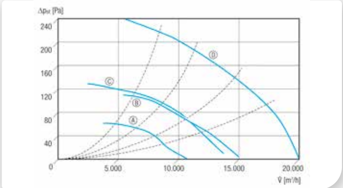
Ⓐ DAS 71/8 Ⓑ DAS 71/6 Ⓒ DAS 80/8 Ⓓ DAS 71/4
