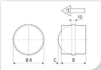
① Förderrichtung
