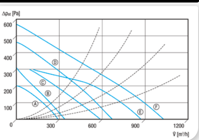
Ⓐ ERM 18 Ex t Ⓑ ERM 18 Ex t/60 Hz Ⓒ ERM 22 Ex t Ⓓ ERM 22 Ex t/60 Hz Ⓔ ERM 25 Ex t Ⓕ ERM 25 Ex t/60 Hz
