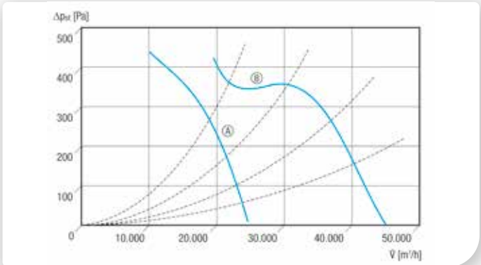
Ⓐ DAD 80/4 Ⓑ DAD 90/4
