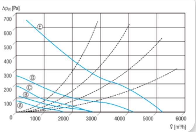
Kennlinien für DN 350 bis DN 400
