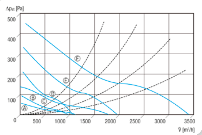
Kennlinien für DN 200 bis DN 300
