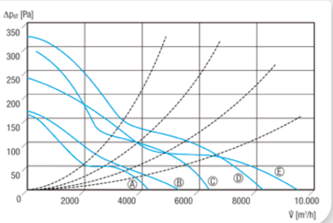
Kennlinien für DN 450, DN 500 und DN 600
