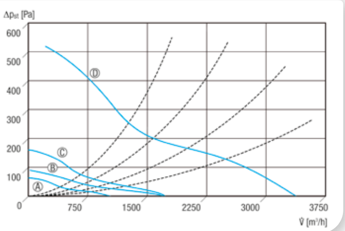
Kennlinien für DN 300 und DN 350
