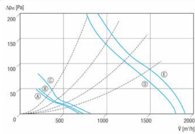
Ⓐ EZD 25/4 E Ⓑ EZD 25/4 D Ⓒ DZD 25/4 D Ⓓ DZD 25/2 B Ⓔ EZD 25/2 B
