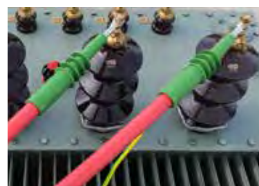
AIP20 als Transformatoranschluss
