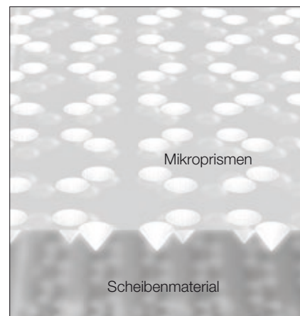
Schnitt durch die TWINDOT Prismenstruktur
