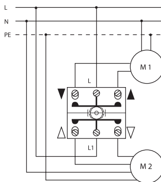
Jalousiedrehschalter/ Schlüsselschalter 2-polig
