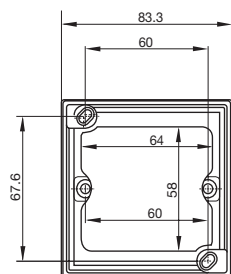
Aufputzgehäuse 1-fach
