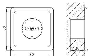
Steckdose 1-fach
