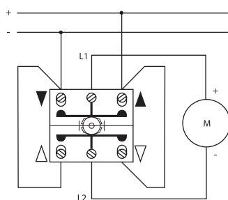
Jalousiedrehschalter, Pol-Wende-Schaltung
