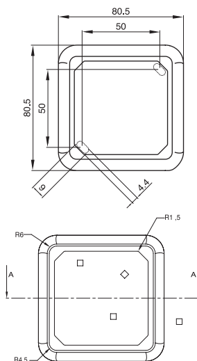
Aufputzgehäuse 1-fach
