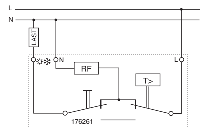
Temperaturregler als Wechsler, Art. 176261
