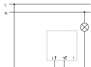
Ausschaltung mit Sensor- oder Tastdimmer
