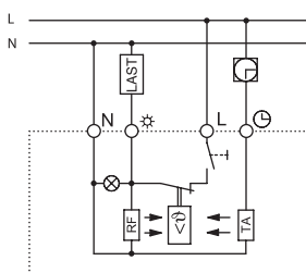
Schaltung als Öffner mit EIN-/AUS-Schalter, Art. 176252
