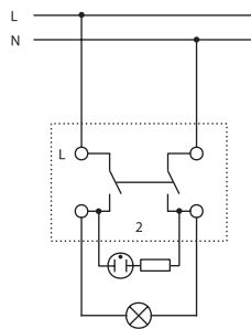
Kontroll-Ausschaltung, 2-polig
