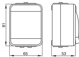
Schalter 1-fach
