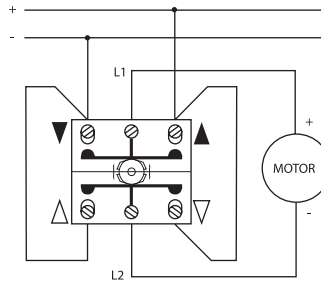
3-Stufenschalter mit 0-Stellung
