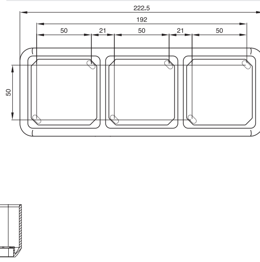
Aufputzgehäuse 3-fach
