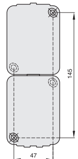
Kombination 2-fach senkrecht
