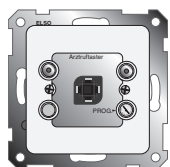
Ruftastereinsatz Arzttruf für FASHION/RIVA/SCALA Einsatz ohne Krallenbefestigung
