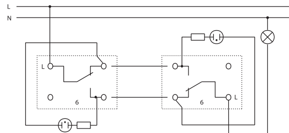
Wechselschaltung
