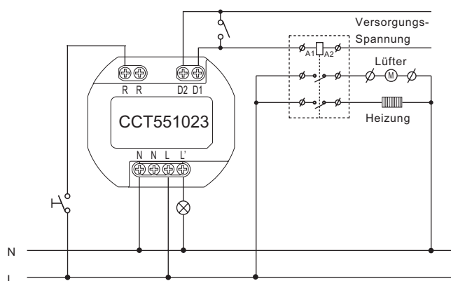
Anschlussbild, Standard-Anwendung
