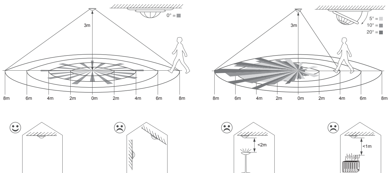
Erfassungsdiagramme
