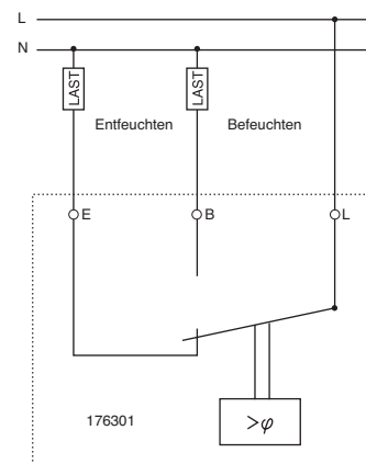
Schaltplan Hygrostat, Art. 176301
