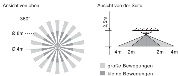
Erfassungsdiagramm
