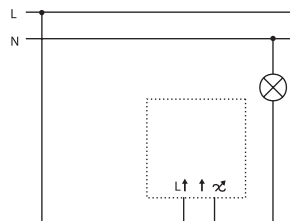
Ausschaltung mit Dimmer Druck-Aus-Wechselschalter
