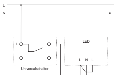
Ausschaltung einfarbiger Einsatz Art. 123209, 123207
