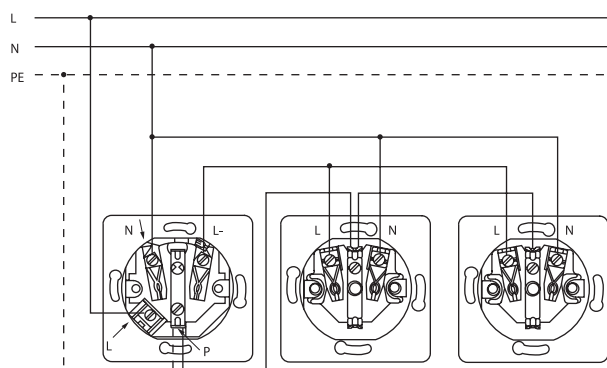
Schaltungsplan
