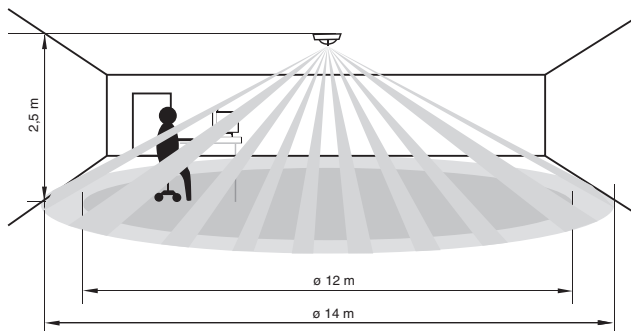
Erfassungsdiagramm
