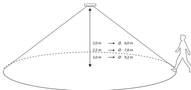
Erfassungsdiagramm
