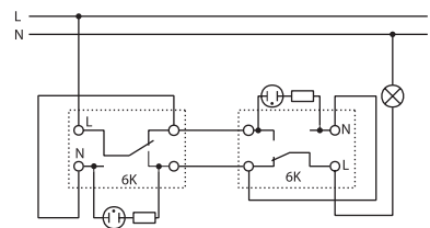
Kontroll-Wechselschaltung/beleuchtet
