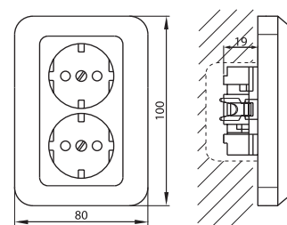
Steckdose 2-fach 1)
