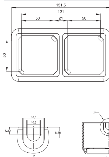
Aufputzgehäuse 2-fach
