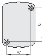
Schalter 1-fach
