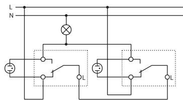
Sparwechselschaltung/beleuchtet
