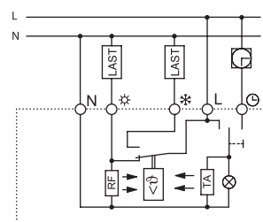
Schaltung als Wechsler mit Wahlschalter, Art. 176232
