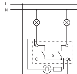
Serienschaltung/beleuchtet mit entsprechender Leuchtmarkierungsbaugruppe
