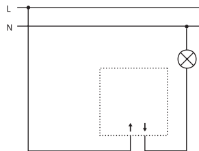
Ausschaltung mit Dimmer Dreh-Ausschalter
