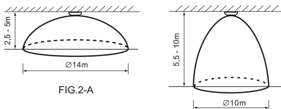
Erfassungsdiagramm
