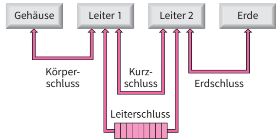
4: Fehlerarten
