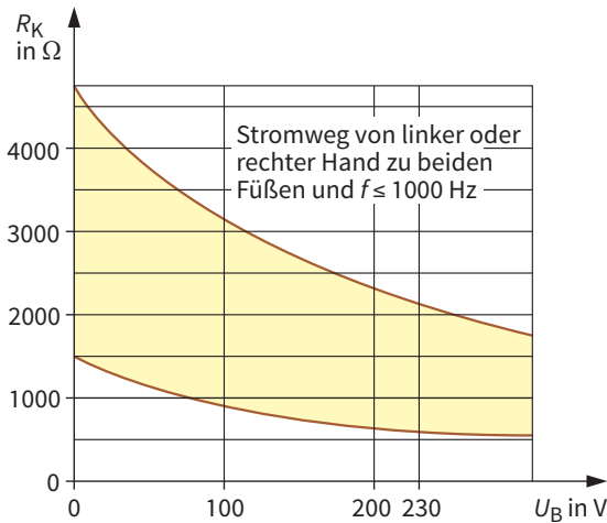
1: Körperwiderstand R_K in Abhängigkeit von U_B (Bereich für mögliche Körperwiderstände)
