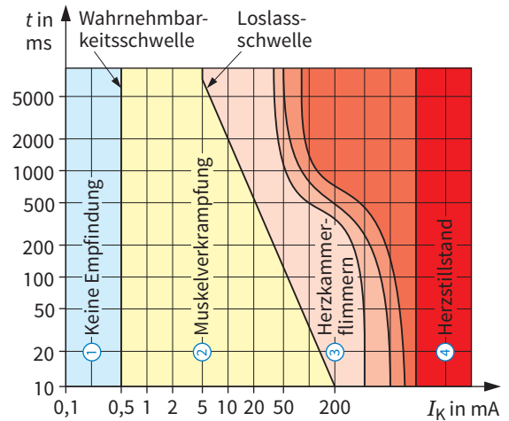
2: Stromstärkebereiche bei Wechselstrom (50 Hz)
