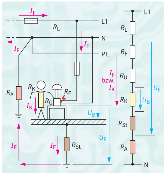
3: Fehlerstromkreis bei Körperschluss
