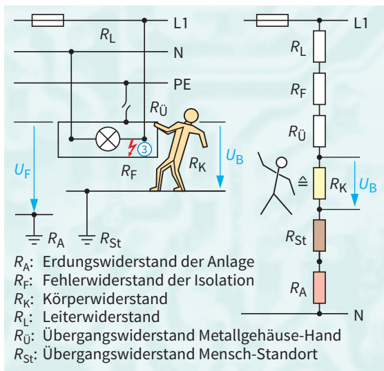
1: Ersatzschaltbilder im Fehlerfall
