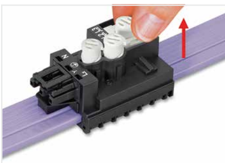
Durch Hochziehen des Drehelementes kann die Arretierung gelöst und durch Schieben der Schalteinheit die neue Phase gewählt werden. Achtung: Nicht an gleicher Stelle der Flachleitung verwenden!
