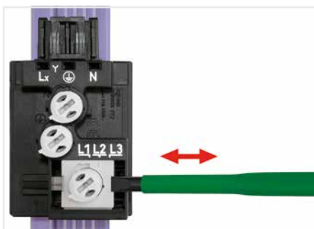
Wahl der gewünschten Phase durch Verschieben der Schalteinheit
