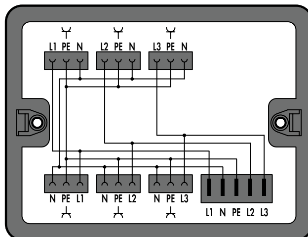
Verteilerbox; Dreh- auf Wechselstrom (400 V/230 V)
