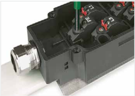
Abgriffmodul mit Leitungsverschraubung aus Messing
