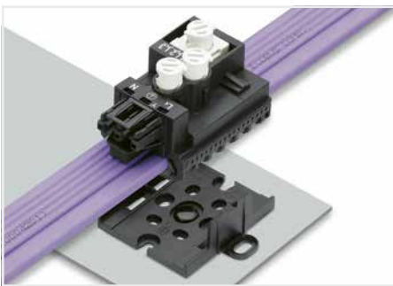
Die Einspeise- und Abgriffmodule verrasten beim Aufstecken auf die Montageplatte.
