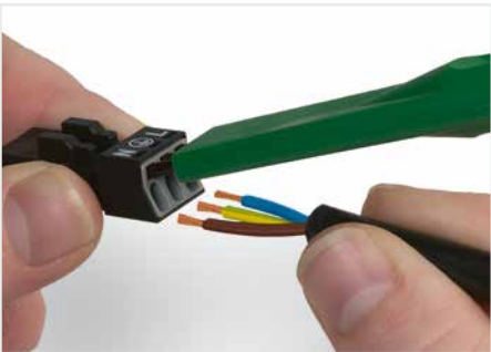
Zum Anschluss feindrähtiger Leiter alle Klemmfedern mittels Betätigungswerkzeug 890-383 öffnen, und abisolierte Leiter bis zum Anschlag einführen.
