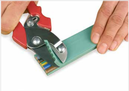
Flachleitungsmantel mit Trennschere abschneiden.
