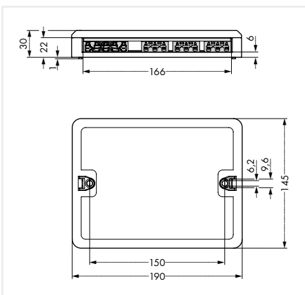
Abmaße einer WINSTA®-Box
