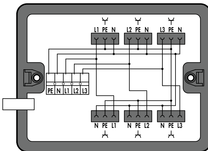
Verteilerbox; Dreh- auf Wechselstrom (400 V/230 V)
