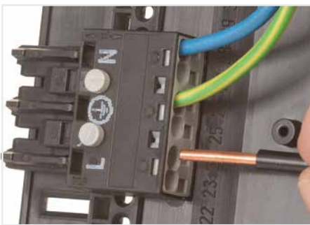
Steckverbinder WINSTA® MIDI können mit Befestigungspins in der Verteilerbox fixiert werden.
