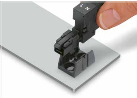
Die Verteiler verrasten beim Aufstecken auf die Montageplatte.
