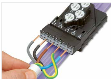
Anschließen einer Mantelleitung an das Einspeisemodul Abisolierte eindrähtige Leiter sind direkt steckbar. Für abisolierte feindrähtige Leiter Klemmstelle vorher mit Schraubendreher öffnen.
