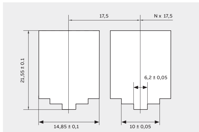
Maße Aussparungen E-DAT-Module
