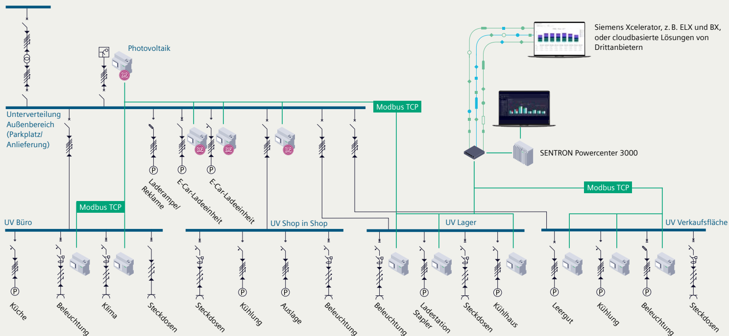
Messgeräte SENTRON 7KM PAC2200
