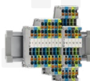
Reihenklemmen mit Push-X-Technologie
