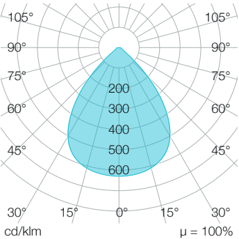
IndustryLUX HEMERA 2.0, 80°
